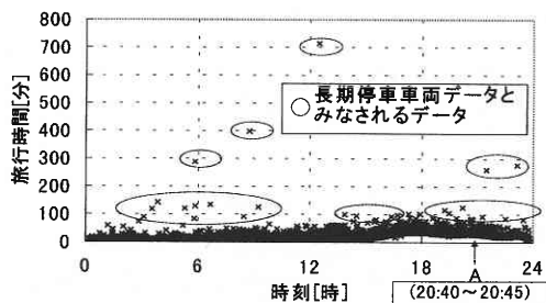
図1 長期停車車両データの例
