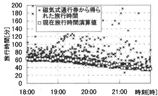
図7 磁気式通行券を利用した現在旅行時間演算結果
