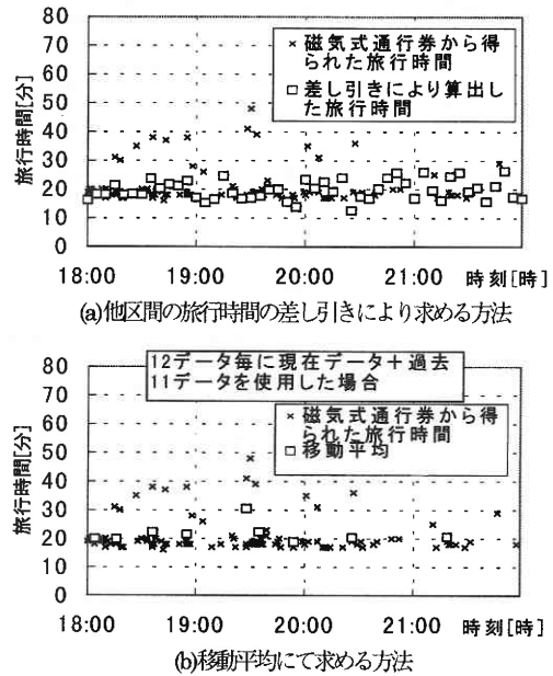
図 11 データ数が少ない場合の対応策
