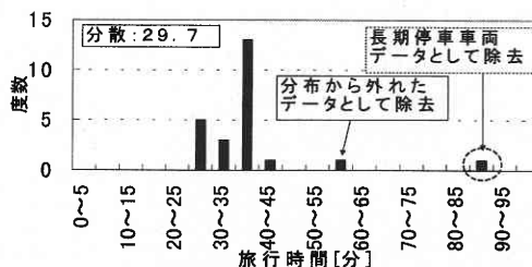
図4 分布から外れた車両データの度数分布例 (5分間蓄積データを使用)
