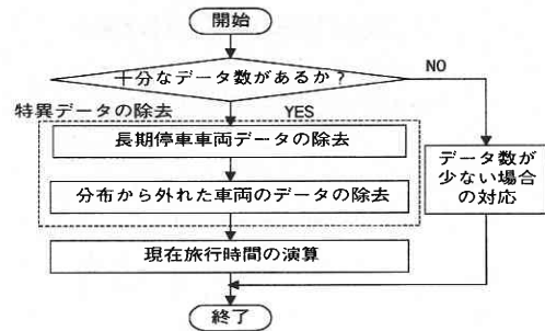
図6 磁気式通行券を利用した現在旅行時間演算方法
