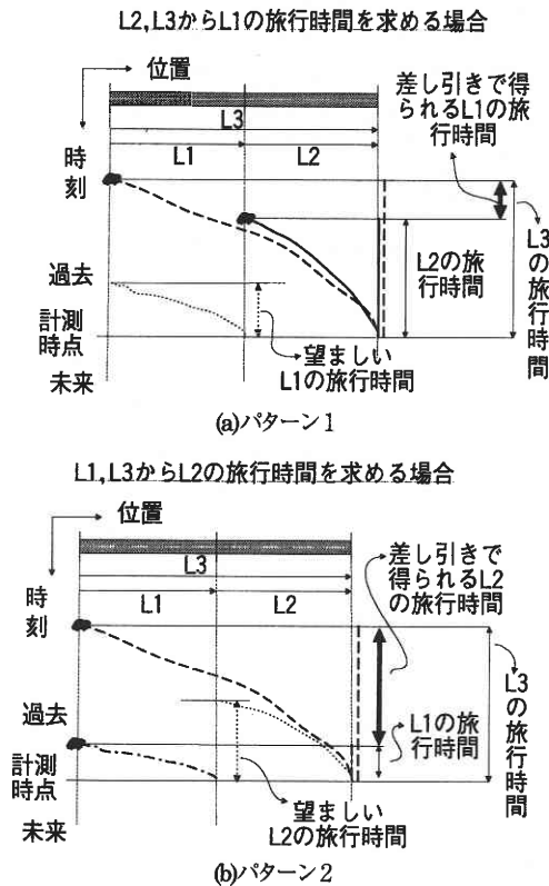
図 10 他区間の旅行時間の差し引きにより求める方法の概念
