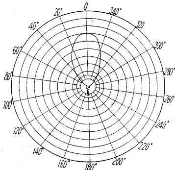
第2図 ヘリカル・アンテナの指向性
