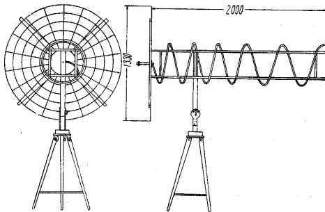
第1図 ヘリカル・アンテナ (225 Mc 受信用)
