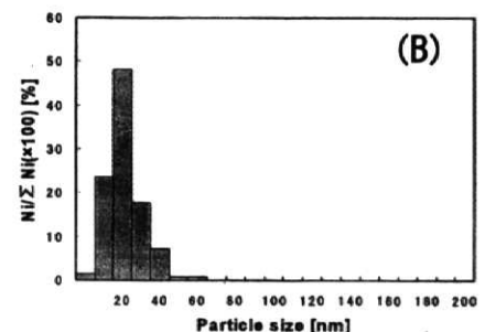
図2 反応時間1分で調製した銀/ \alpha -アルミナ；(A) TEM像、(B) 銀微粒子の粒度分布
