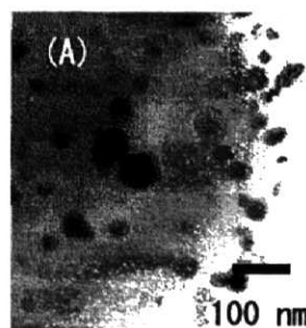
図2 反応時間1分で調製した銀/ \alpha -アルミナ；(A) TEM像、(B) 銀微粒子の粒度分布
