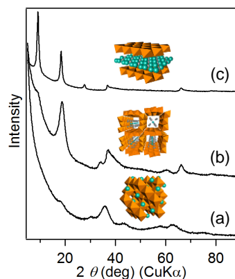
Figure 4. Co-Mn 酸化物合成時の水量を変化させた際の生成物の XRD パターン (H 2 O/Co = (a) 0, (b) 20, (c) 60 (mol/mol)).
