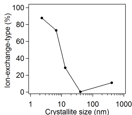
Figure 5. 異なる粒径を有する Li-Mn スピネル酸化物からの Li + の脱離の際のイオン交換型の反応の割合.
