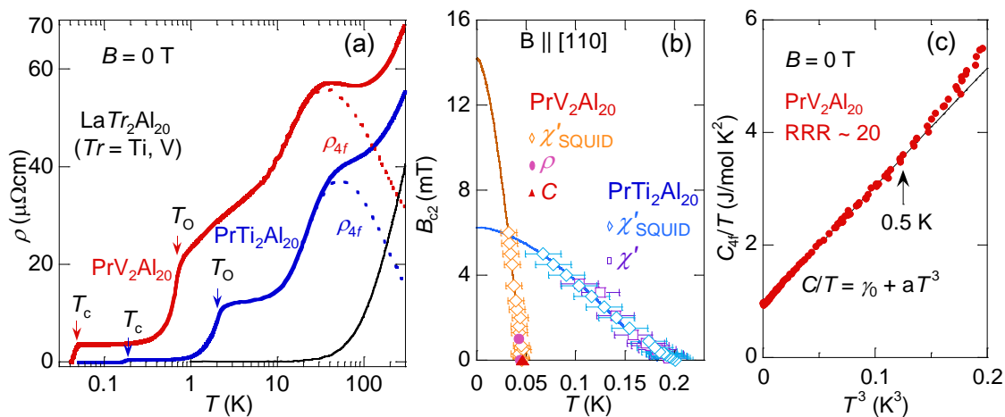
図 1. (a) \text{PrTi}_2\text{Al}_{20} , \text{PrV}_2\text{Al}_{20} の電気抵抗率の温度依存性。本研究で \text{PrV}_2\text{Al}_{20} の四極子秩序状態において 0.05 \text{ K} で超伝導が実現した。(b) 超伝導の温度—磁場相図。実線は WHH フィッティングの結果を表す。 \text{PrV}_2\text{Al}_{20} の超伝導は常圧下において \text{PrTi}_2\text{Al}_{20} よりも磁場に対して鈍感で、準粒子の有効質量が大きい重い電子超伝導状態となっている。(c) 比熱は四極子秩序状態において T^4 に比例する。切片は非常に大きく、 \gamma が 0.9 \text{ J/mol K}^2 にも達する。
