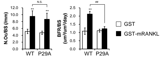
Fig. 1 P29A ホモ変異マウスでは骨吸収と骨形成のカップリングが抑制されている
