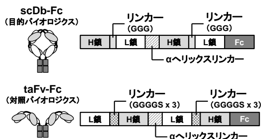
Fig. 4 各バイオロジクスの構造
