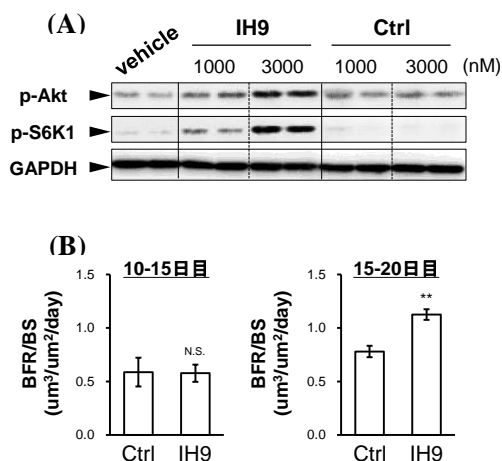
Fig. 3 IH9 scFv 二量体は生体内で骨形成を促進する作用を有する
