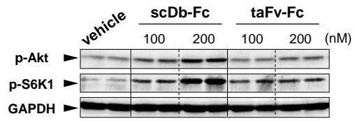
Fig. 5 scDb-Fc は低濃度から RANKL 逆シグナルを活性化するのに対し、taFv-Fc はシグナル入力活性をほとんど示さない
