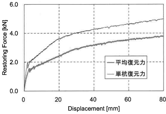
図12 復元力-変位履歴
