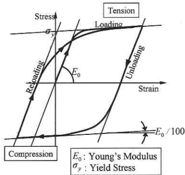
図4 鉄筋モデル
