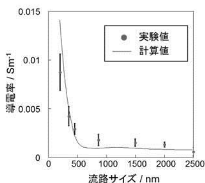
図7 導電率の流路サイズ依存性 (試料: 純水)
