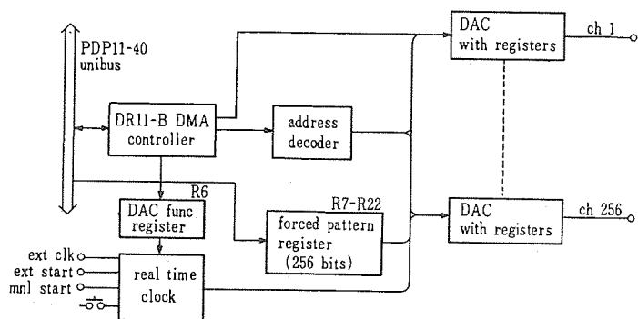
第 1 図 多点同時刺激装置
