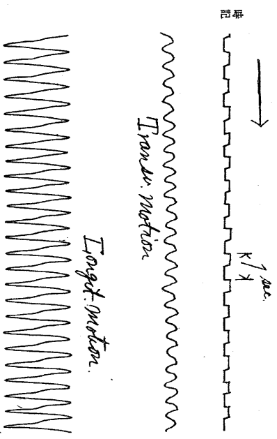
第五十九圖 瓦斯機關三臺運轉ス (相差前位相ノ差ヲ百二十度トス) 大正四年二月十八日機關地盤中央ニテ記錄ス
