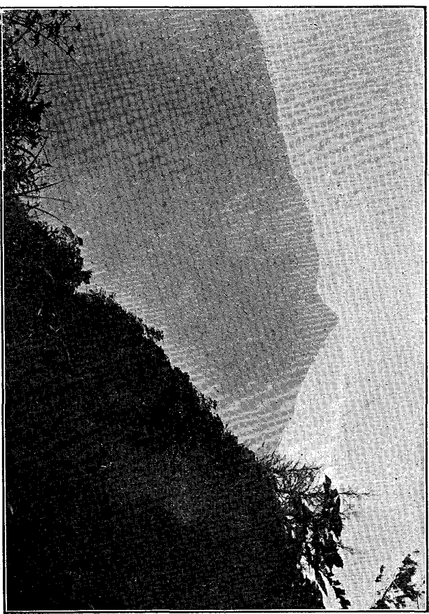
嶽ノ經ハドツミラビノ中央、ム望ヲ嶽ノ經ニ北東リヨ腹山南ノ木黒 圖三第 。リテ上頂ノ
