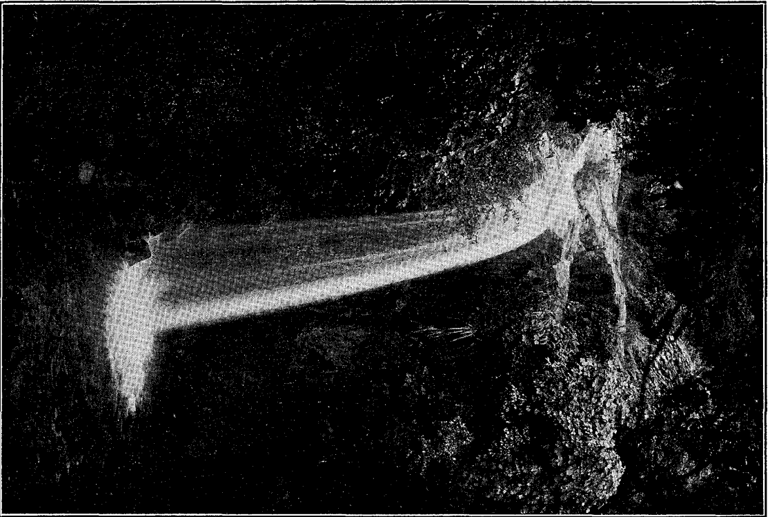
Fig. 2. Ayngayeri waterfall.
