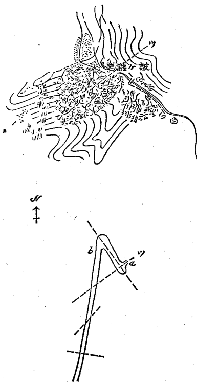
鼓ノ瀧ノ裂罅線圖 (圖四第)
