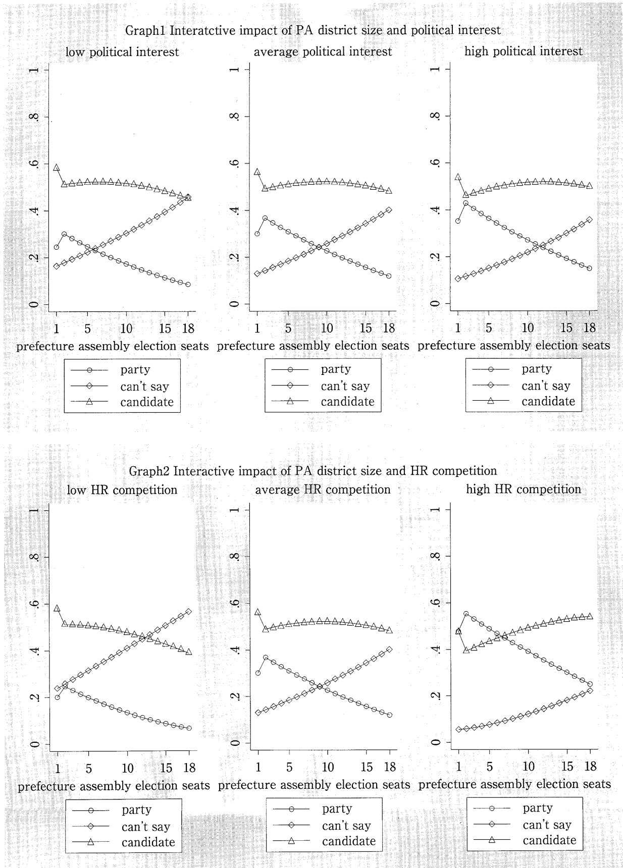
図1 予測確率
