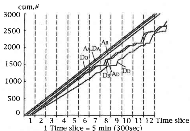
図6 実験ネットワークによる累積交通量図
