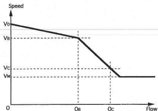
図7 COBA型Q-V曲線
