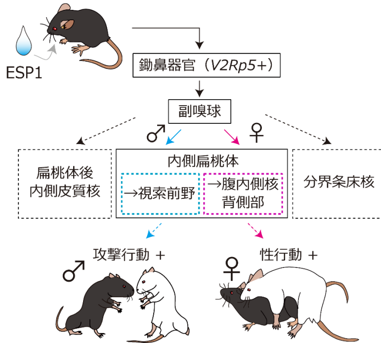
図) ESP1 によるフェロモン誘発行動を制御する神経基盤の概要
