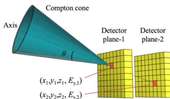
図1：コンプトンイメージングシステム概念図
