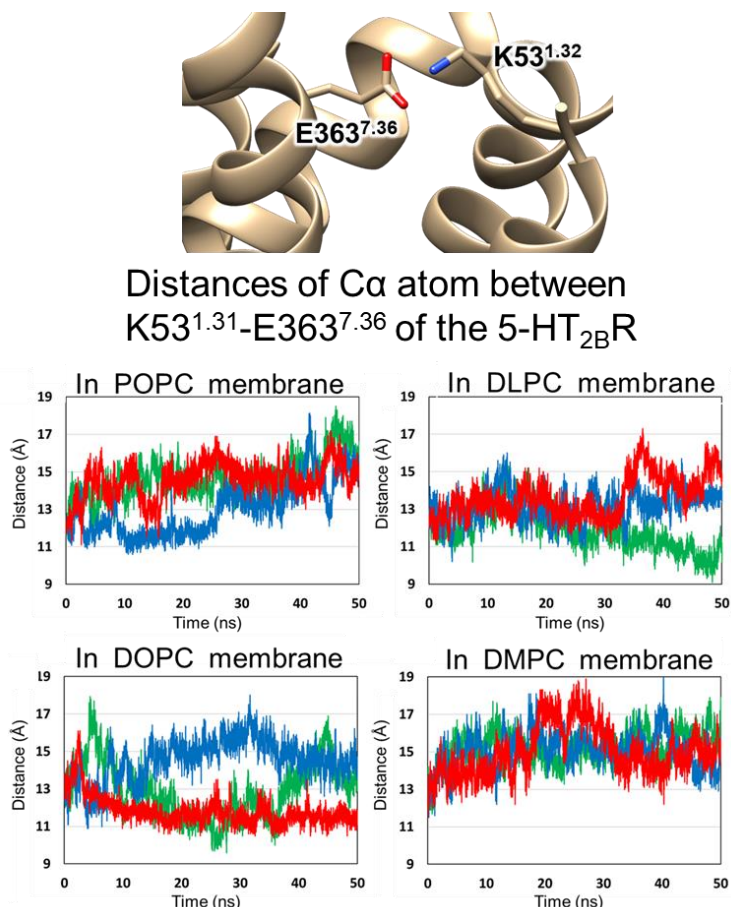
図 4. TM1-TM7 間の静電的相互作用形成
