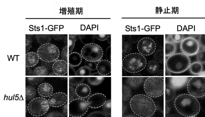
図4A. Sts1は静止期にHul5依存的に粒状構造体を形成する
