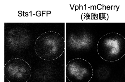
図4B. Sts1は静止期に液胞に局在する
