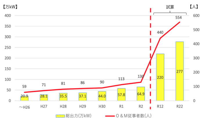
図3 秋田県の風力発電の導入状況と O&M 従事者数
