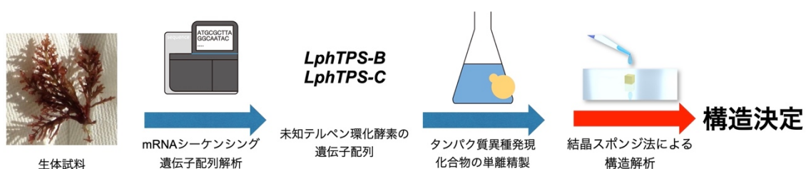
図3 本研究が提唱する、CS法を組み込んだ遺伝子情報に基づく生合成研究のワークフロー。NMRやMSに先立ってCS法による構造解析を行い、実験系のスケールダウンや構造解析の迅速化を狙った。
