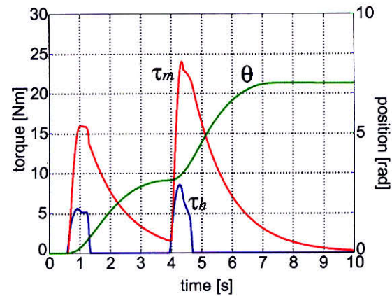
(b) 左輪トルクと位置応答
