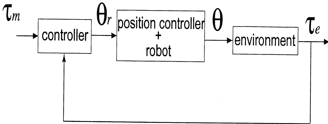
図 3.2: 位置制御ベース型パワーアシスト法の基本構成図
