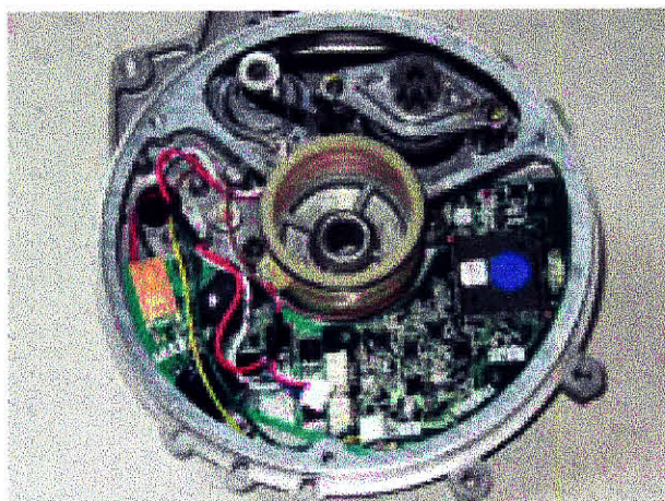
図 D.7: JWII の基板
