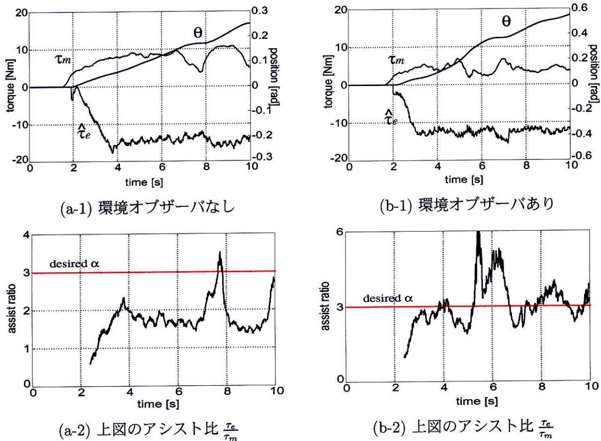
図 3.36: K_e = 800 として段ボールを押した実験結果
