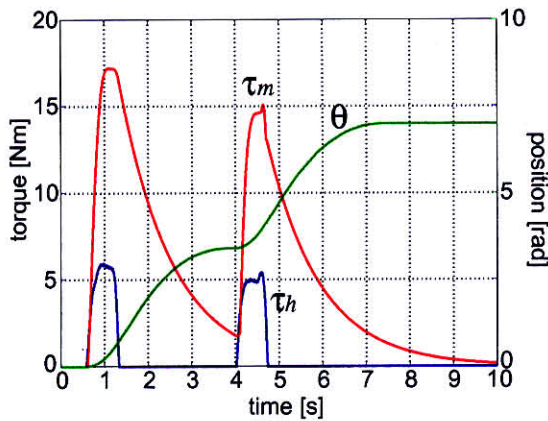
(a) 右輪トルクと位置応答
