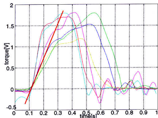
(b) 後方へ転倒した際の操作者入力トルク
