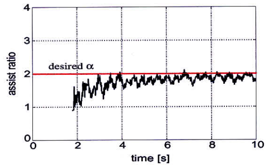
(b-2) 左図のアシスト比 \frac{\tau_e}{\tau_m}
