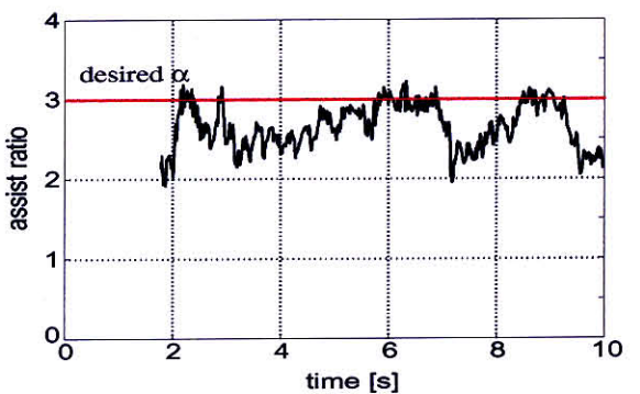
(b-2) 左図のアシスト比 \frac{\tau_e}{\tau_m}
