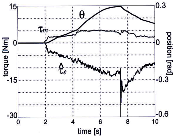
(b-1) 位置と力の応答
