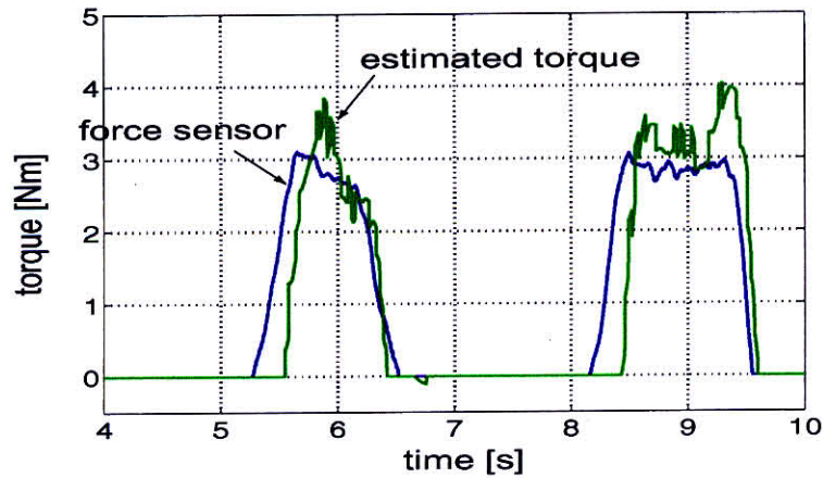
図 4.2: 操作者の入力トルクの推定
