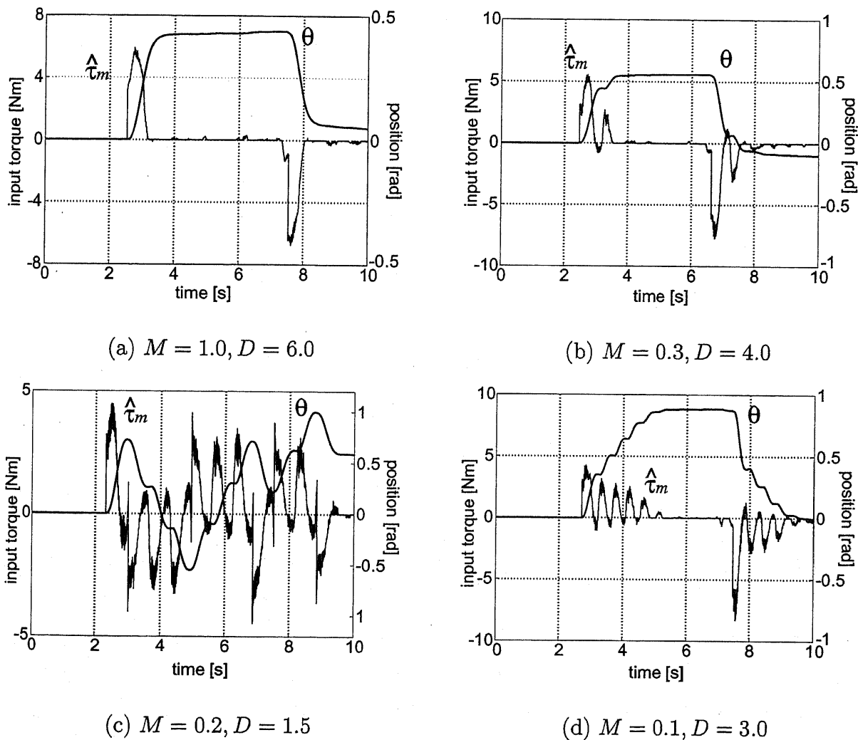
図 4.20: 慣性変動した際のセンサレスインピーダンス制御 ( J_n = 0.44 )
