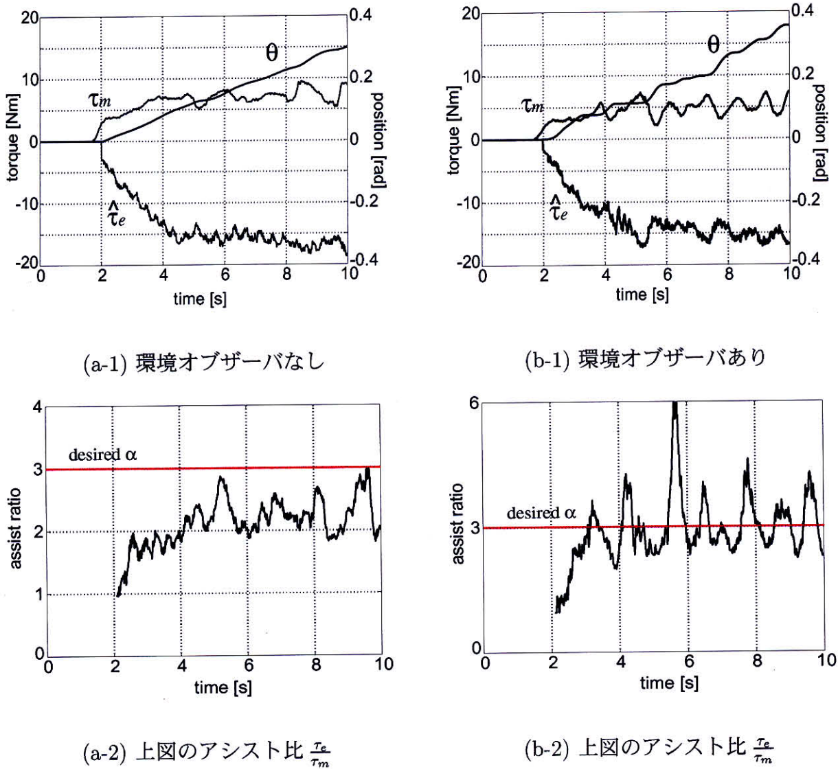
図 3.38: D_e = 10 , K_e = 400 として段ボールを押した実験結果
