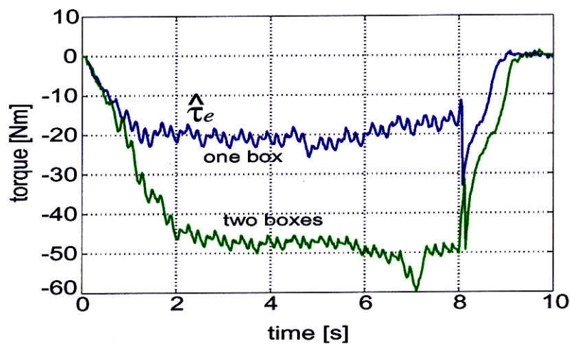
図 3.50: 段ボールを押すために必要な環境作用力の推定
