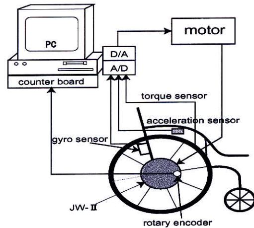
(b) 実験機の構成
