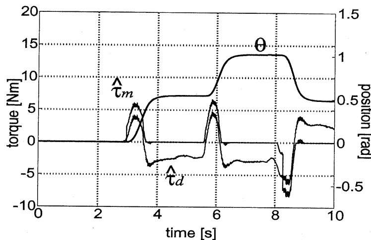
図 4.4: センサレスインピーダンス制御の実現
