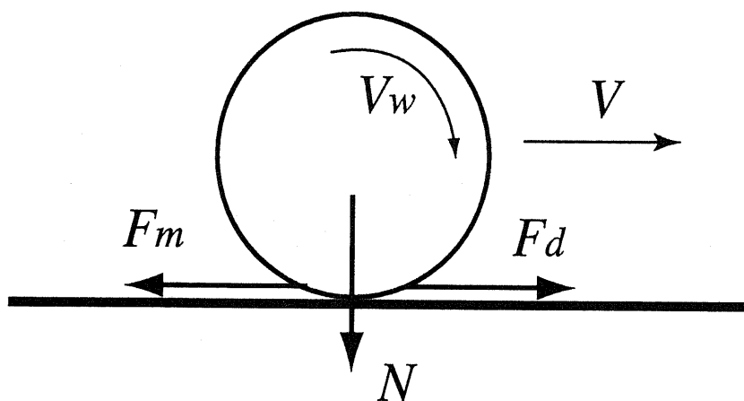
図 5.7: 車椅子の一輪モデル
