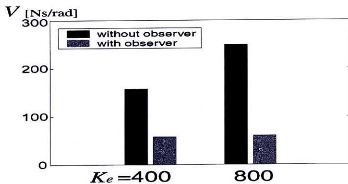
図 3.37: 環境オブザーバの効果
