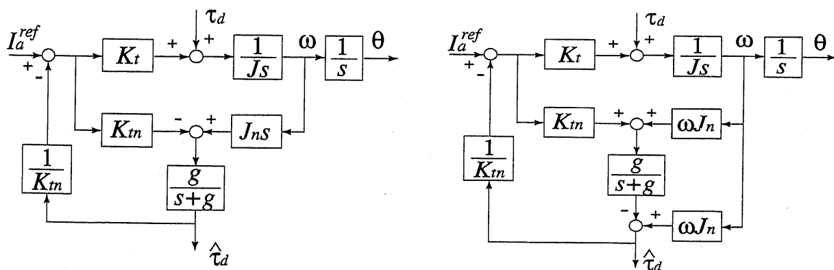
(a) 速度情報に基づく外乱オブザーバの基本構成
