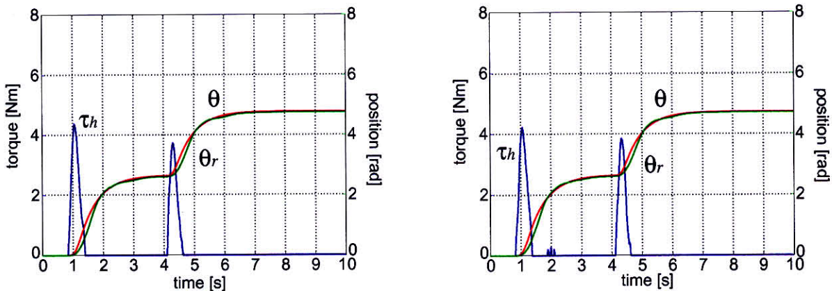
(b) 左入力トルクと位置応答
