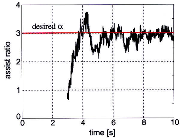
(b-2) 上図のアシスト比 \frac{\tau_e}{\tau_m}
