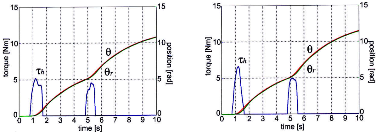
(b) 左入力カトルクと位置応答
