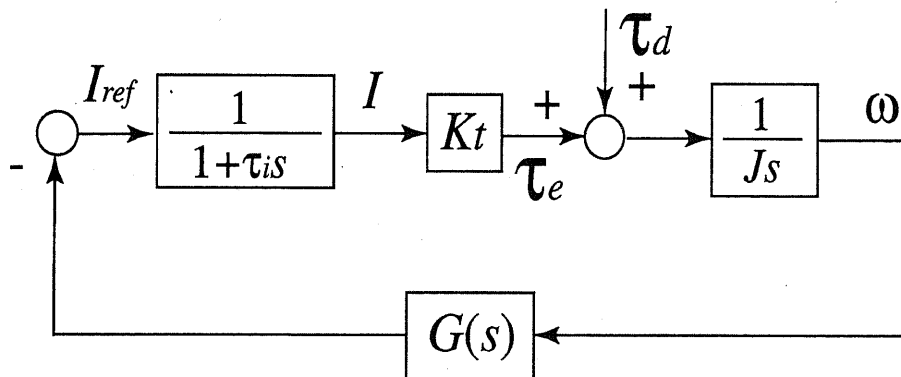
図 6.16: 慣性制御系の構成
