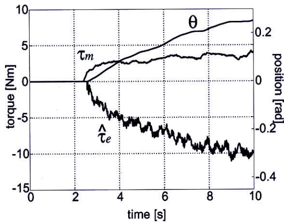
(b-1) Q = 3 としたときの位置と力の応答
