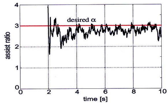
(a-2) 左図のアシスト比 \frac{\tau_e}{\tau_m}
