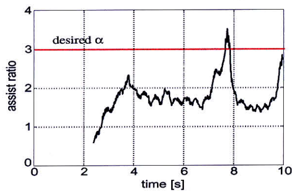
(e-2) 左図のアシスト比 \frac{\tau_e}{\tau_m}
