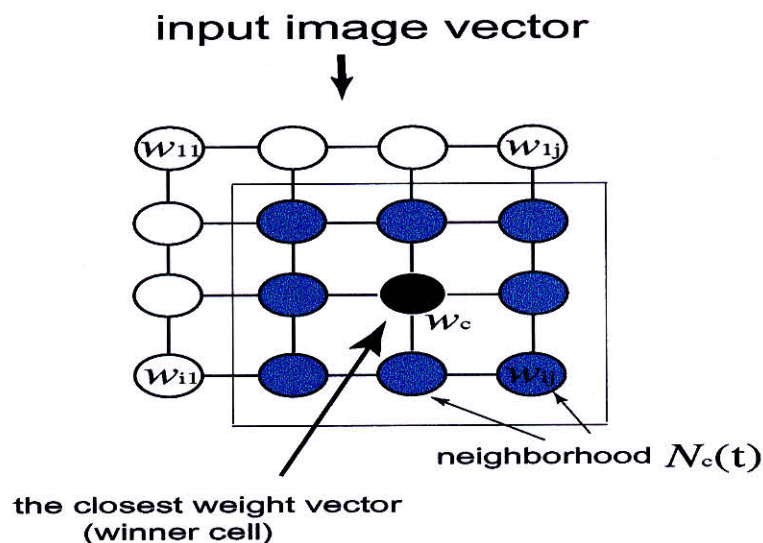
図 8.7: 2次元自己組織化マップ
