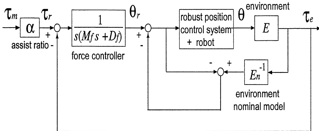
図 3.30: 環境オブザーバを用いたパワーアシスト制御系
