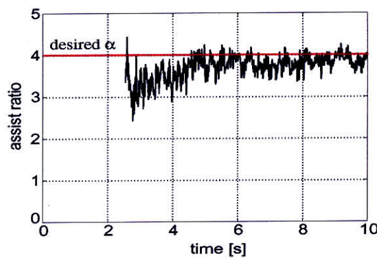
(c-2) 左図のアシスト比 \frac{\tau_e}{\tau_m}
