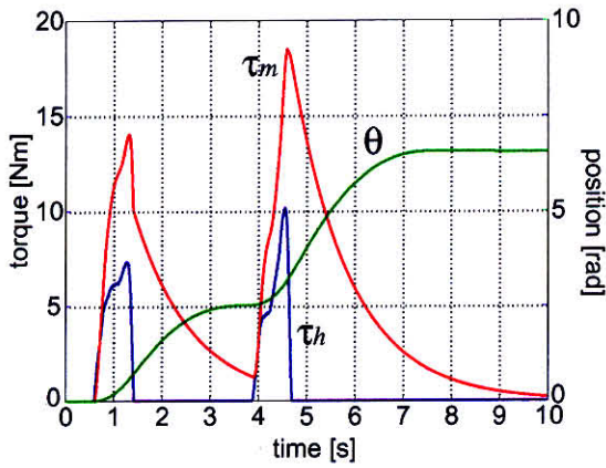
(a) 右輪トルクと位置応答
