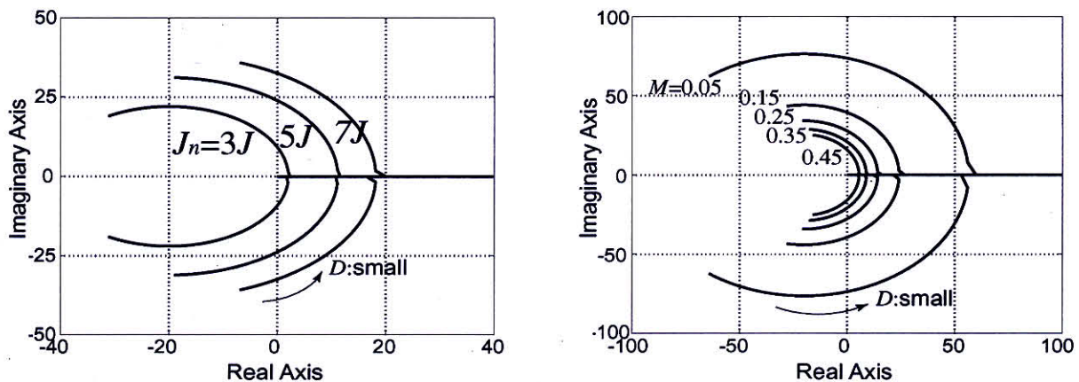
(a) 慣性変動の大きさの影響
