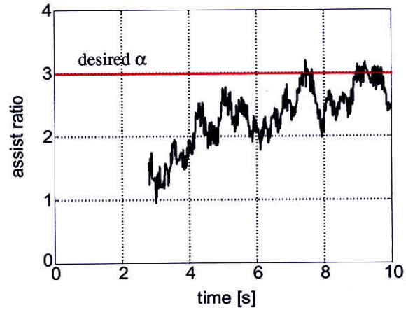
(b-2) 左図のアシスト比 \frac{\tau_e}{\tau_m}
