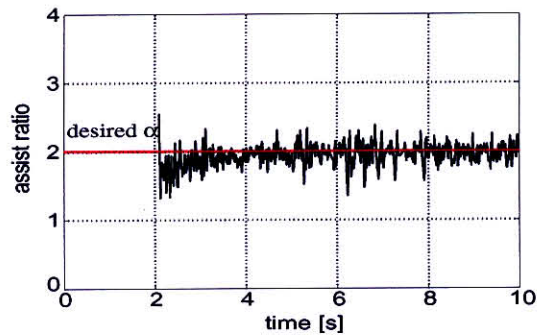
(a-2) 左図のアシスト比 \frac{\tau_e}{\tau_m}
