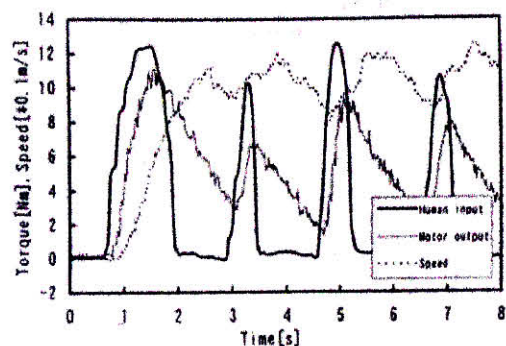
(b) 人間の入力トルクとモータ出力、速度
