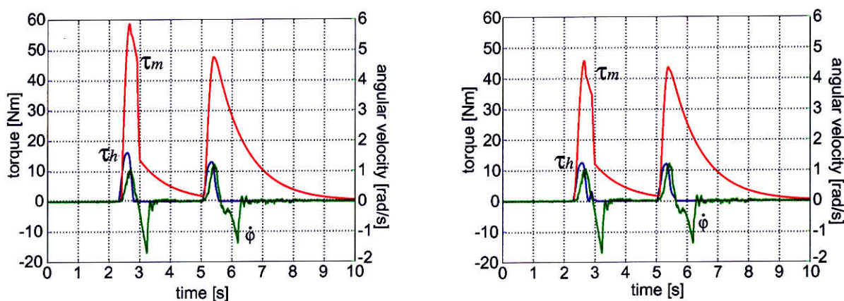
(b) 左輪トルクと浮上角速度
