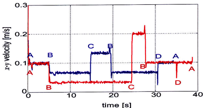
図 9.20: x - y 平面における速度
