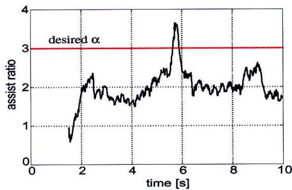
(d-2) 左図のアシスト比 \frac{\tau_e}{\tau_m}
