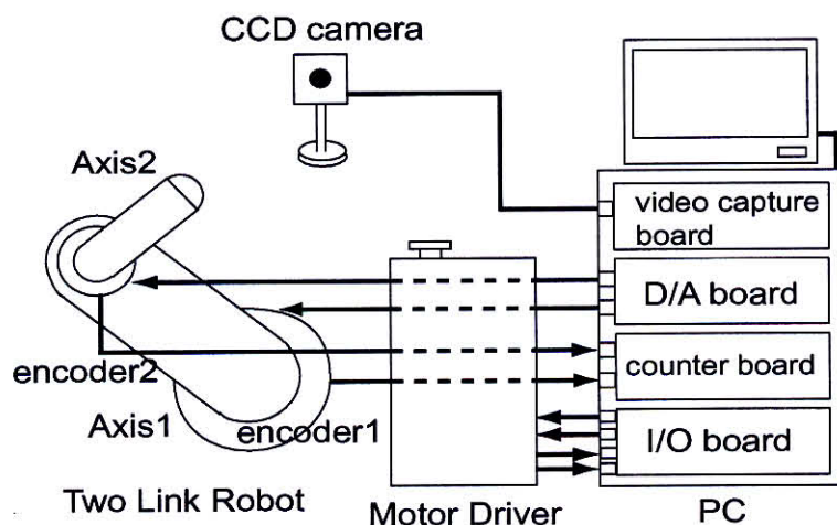
図 9.3: 実験装置の構成
