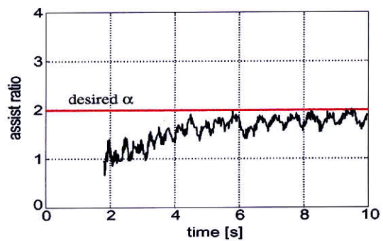
(c-2) 左図のアシスト比 \frac{\tau_e}{\tau_m}
