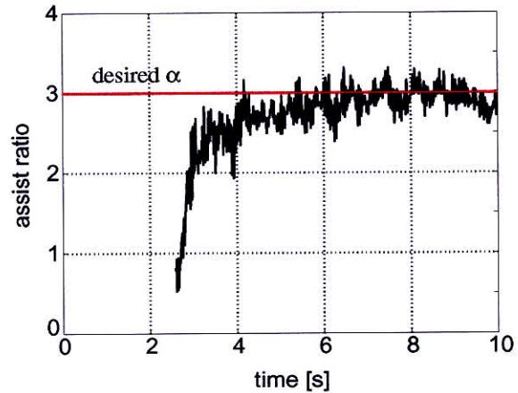
(b-1) 環境オブザーバあり
