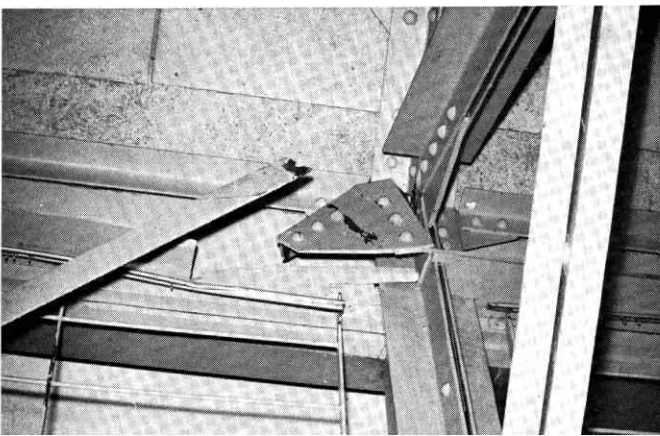
㉓八戸高体育館 —桁行方向のブレースが破断した—
