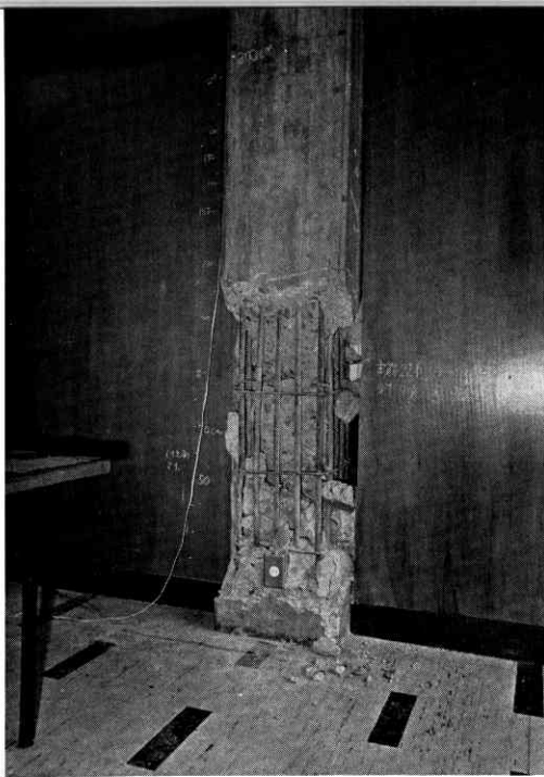
⑳八戸市立図書館
