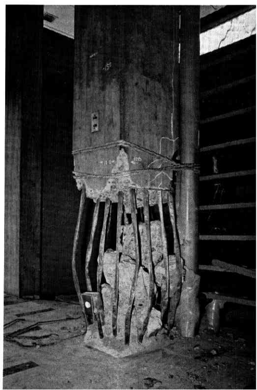
⑲八戸市立図書館 —柱脚が大破壊した—
