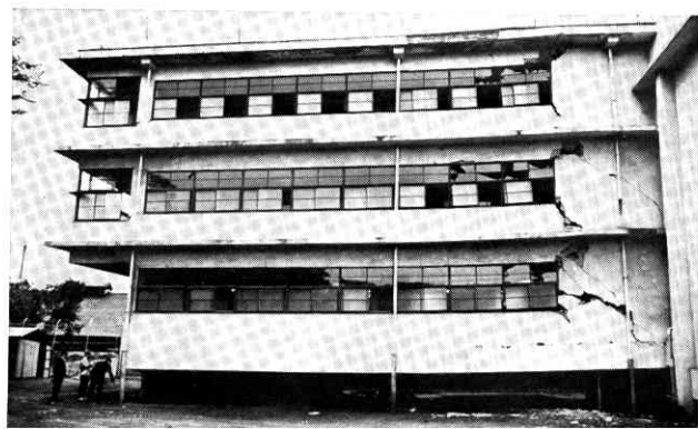
⑯八戸東高 —建物の一部の不同沈下および地下柱の崩壊により左方へ大きく傾いた—
