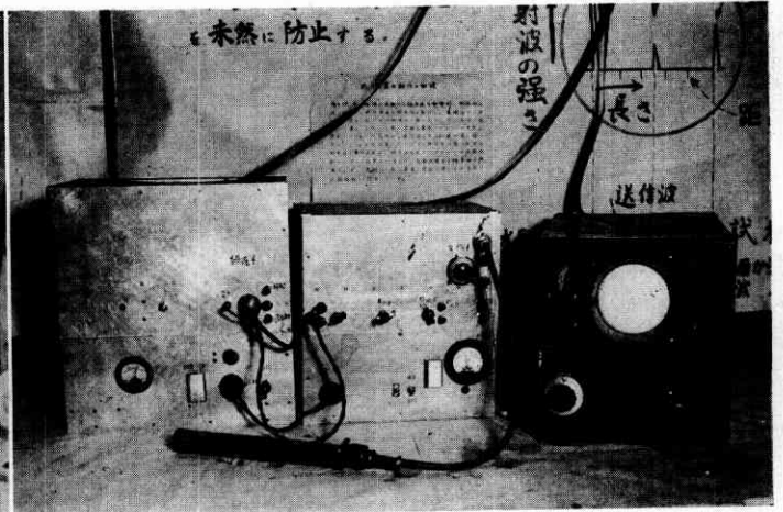
② レーダー方式で材料内の見えない傷を探知する超音波探傷器
