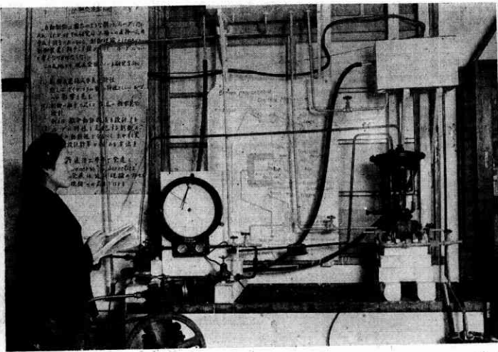
③ 空気作動温度制御装置 (機械 高橋研究室)
