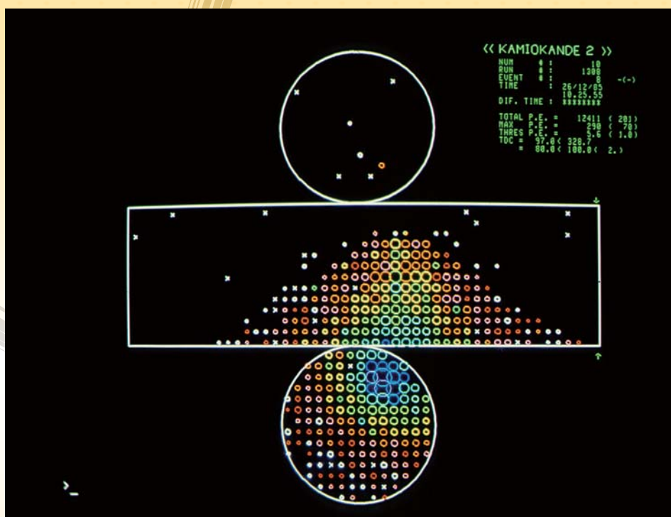
カミオカンデでとらえた宇宙線ミュー粒子事象
