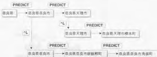
図4.7: PREDICTによる候補空間の採策
