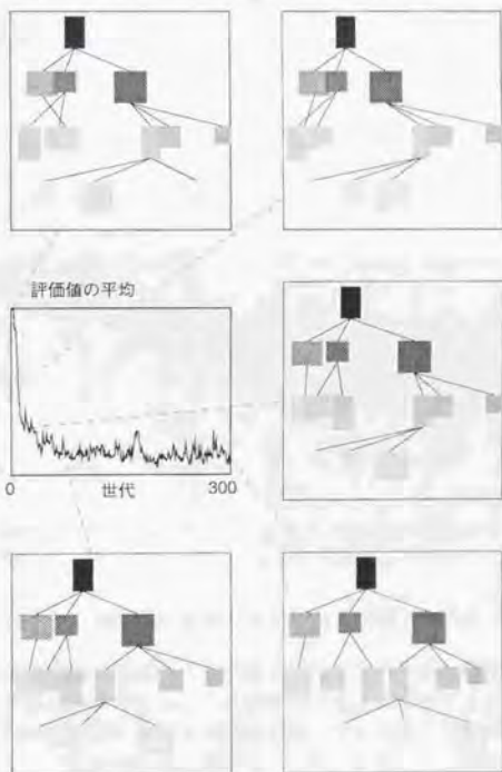
図 6.3: 木構造の配置への遺伝的アルゴリズムの適用
