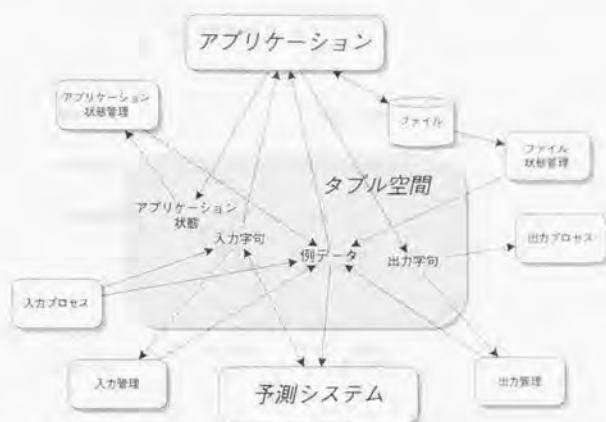
図 7.19: 共有空間通信で実現した統合的予測 / 例示インタフェースアーキテクチャ
