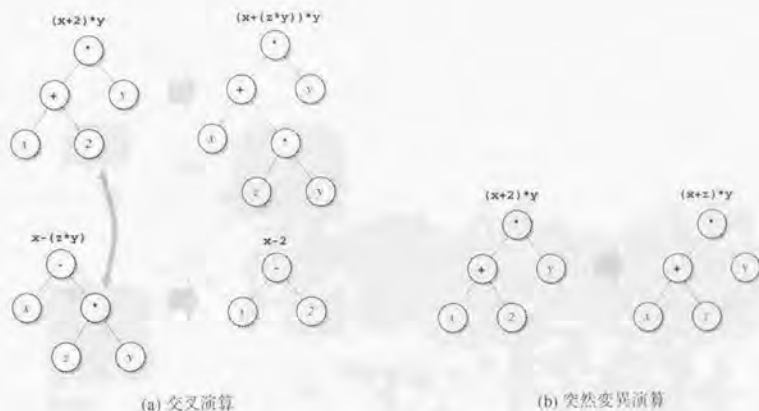
図 6.17: 遺伝的プログラミングの遺伝的演算
