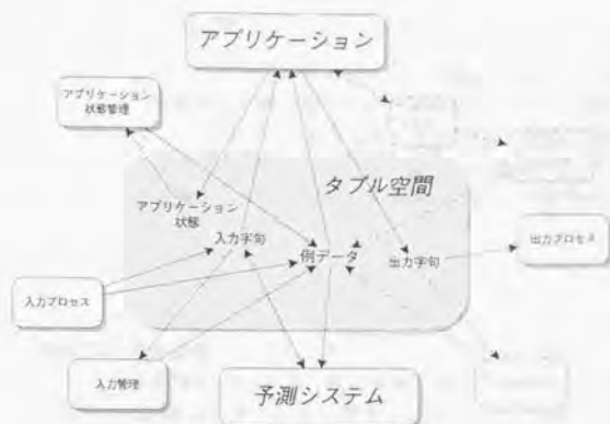
図 7.23: 図形配置評価関数獲得システムの実現
