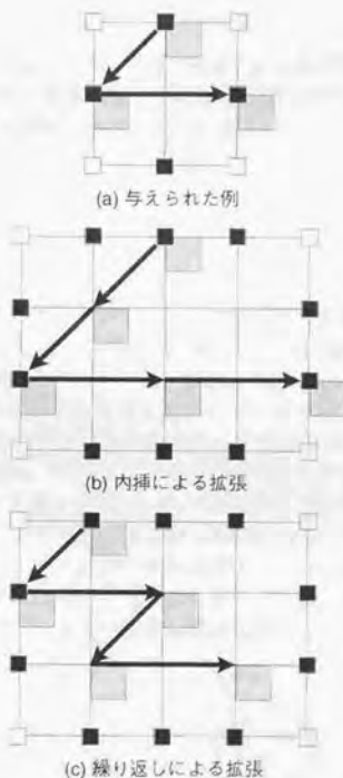
図 2.15: Layout by Example における推論
