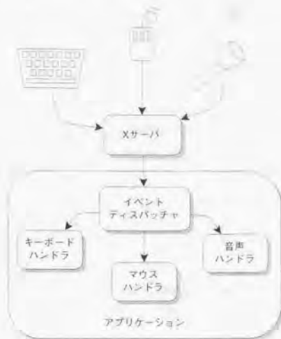
図 7.1: X ウィンドウシステムのイベント処理
