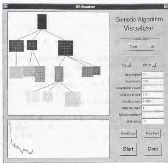
図 6.14: GA ビジュアライザ
