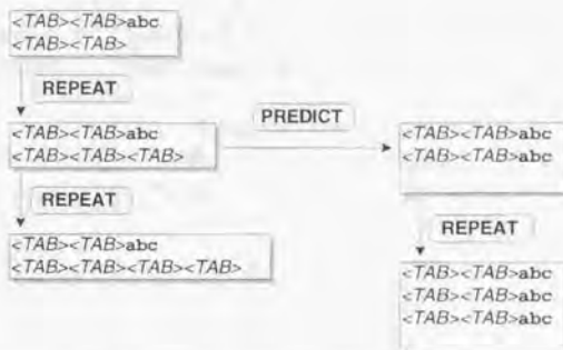
図 4.9: PREDICTによる予測手法の切り替え (1)
