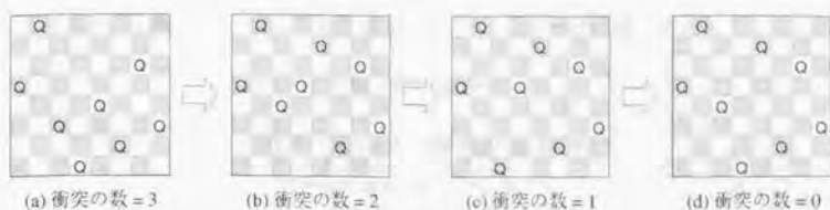
図 6.2: 8-Queen 問題への遺伝的アルゴリズムの適用
