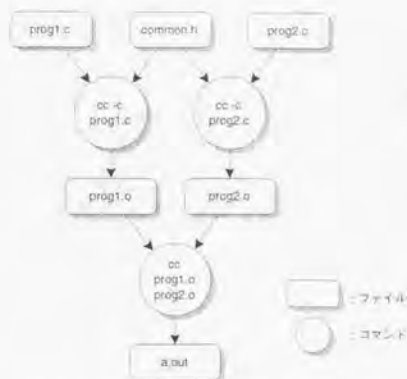
図 5.1: ファイルの依存関係を示すグラフ
