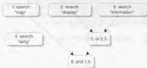
図 5.7: 検索コマンド間の依存関係
