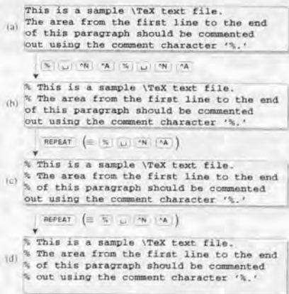
図 4.2: 各行の先頭に注釈記号を追加(2)
