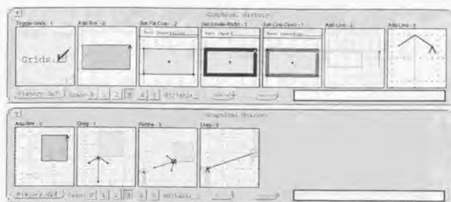
図 2.11: Chimera における図 2.10 の操作履歴のグラフィカル表現
