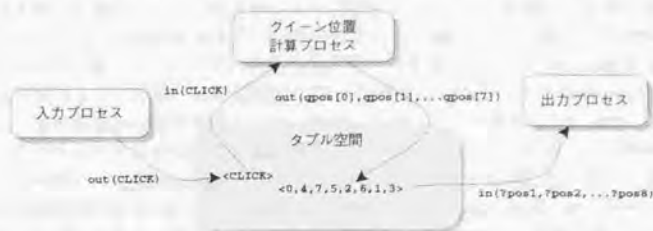
図 7.8: 8-Queen 問題におけるタブル交換
