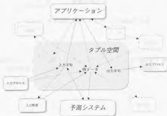
図 7.20: 共有空間通信による Dynamic Macro の実現
