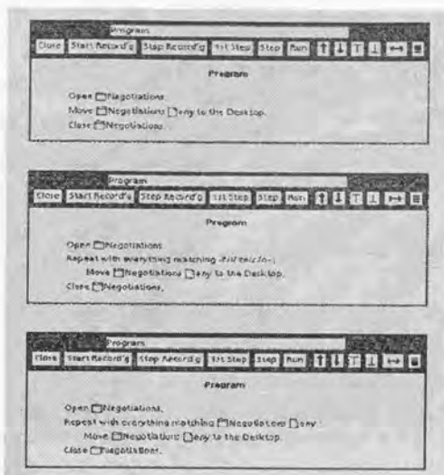
図 2.9: 編集により修正が加えられたプログラム
