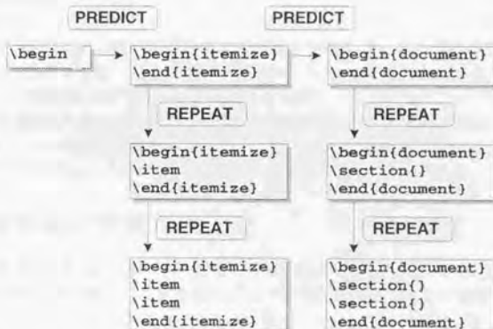
図 4.12: L A T E X プリミティブの予測
