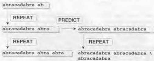
図 4.10: PREDICTによる予測手法の切り替え (2)
