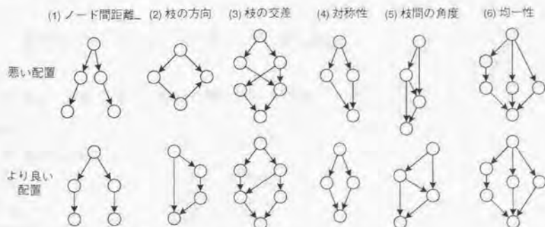
図 6.11: 有向グラフの配置における制約
