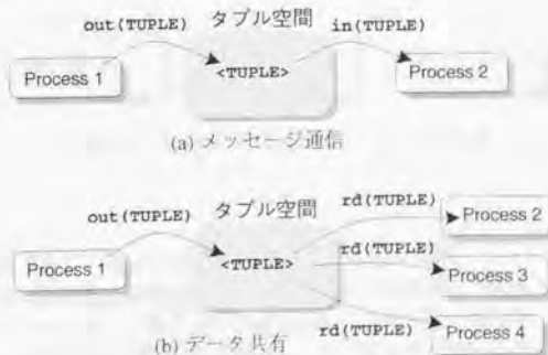
図7.3: タプル空間を使った通信
