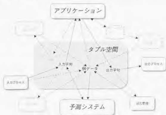
図 7.24: 共有空間通信による Triggers システムの実現
