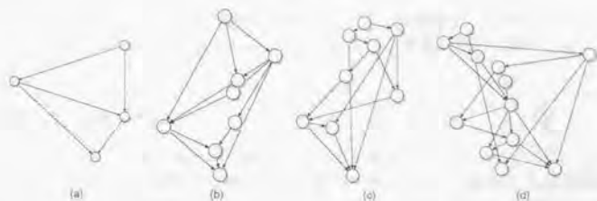
図 6.22: f_b を用いて計算した配置結果
