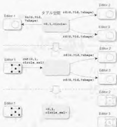
図7.14: 図形の選択時におけるタブの交換
