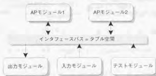
図7.4: タブル空間によるモジュールの分離
