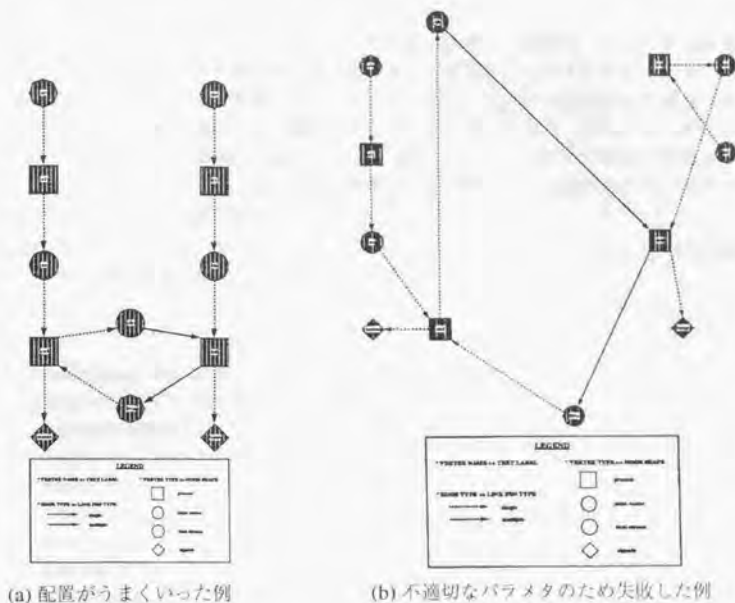
図 6.12: Kosak のシステムによる配置の実行例 ([36]による)
