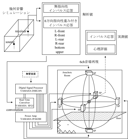
Fig. 1 幾何音響シミュレーションに基づく6チャンネル音場再現システム
