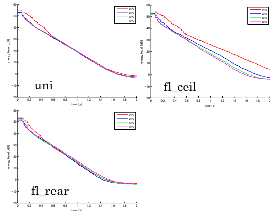
Fig. 5 残響減衰曲線(受音点1、1kHz)
