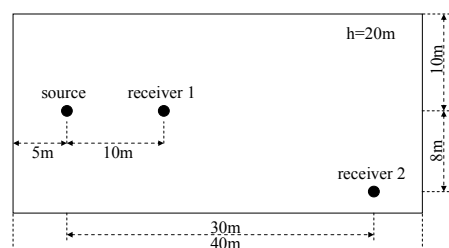
Fig. 2 音源と受信点の位置関係（平面図）
