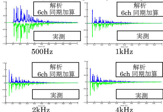
Fig. 4 RMS時間波形 (uni_sc20, 受音点1)
