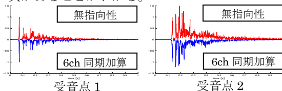
Fig. 3 RMS時間波形 (uni_sc20, 1kHz)
