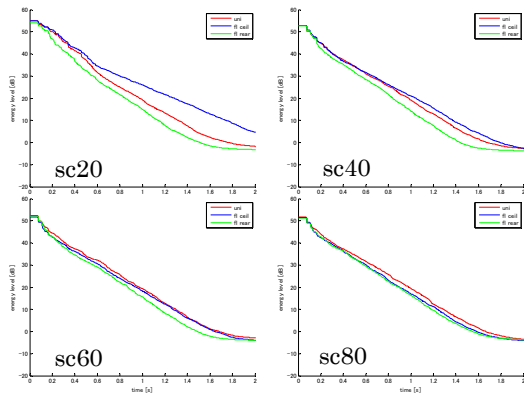
Fig. 6 残響減衰曲線 (受音点 1, 1kHz)
