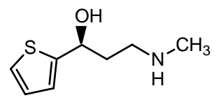
(S)-3
