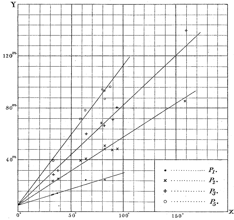
Fig. 2, a. Alasca earthquake:
