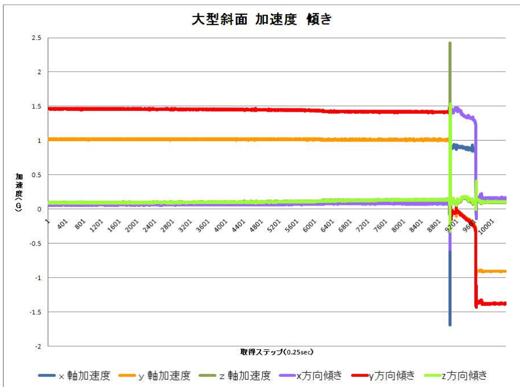
図 4.20 単独杭大型斜面実験において取得した加速度と傾き
