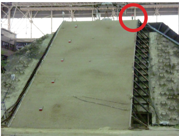
図 4.17 単独杭大型斜面実験杭の設置場所
