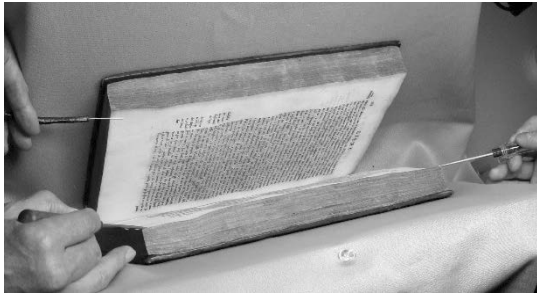
写真 4 あおり撮影の装置
