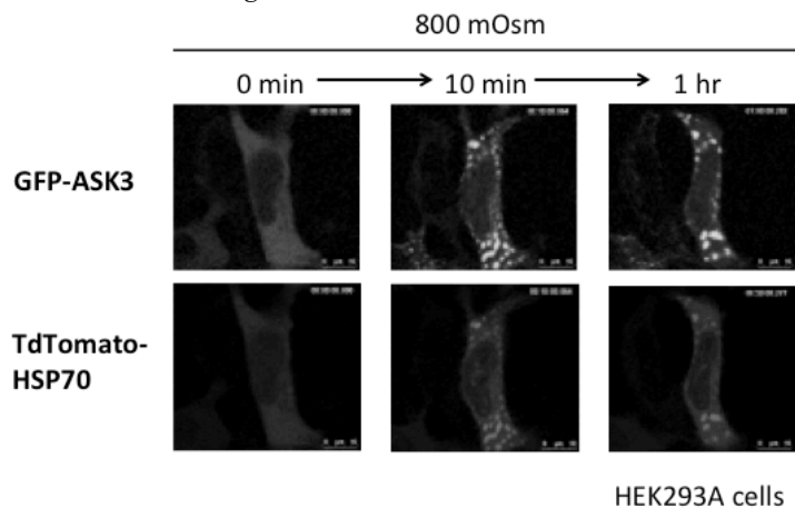
図2 ASK3とHSP70は高浸透圧でグラニューール状に共局在する
