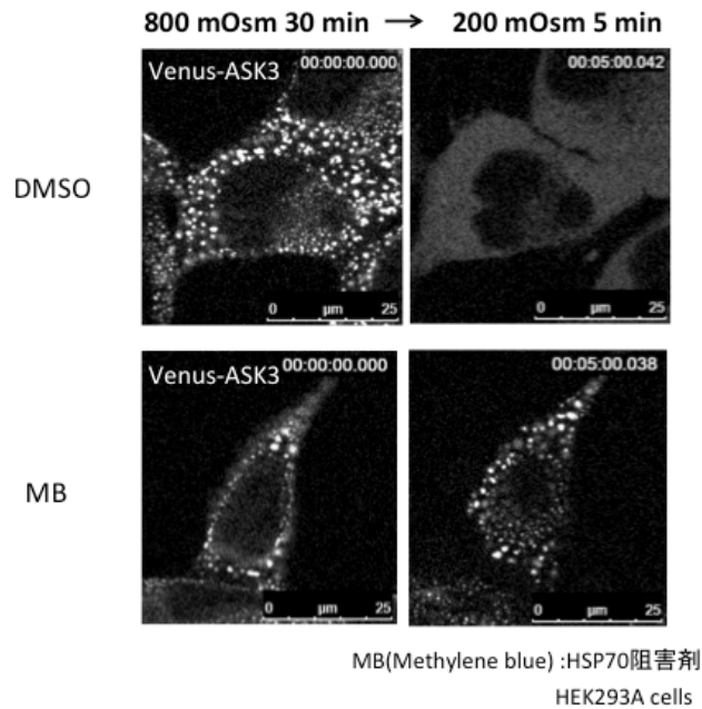
図4 HSP70の阻害によりASK3グラニュールの可逆性が失われる
