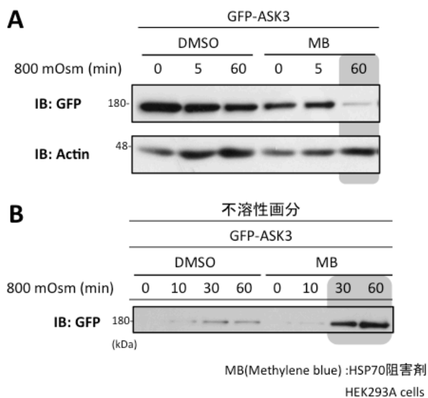
図3 HSP70の阻害は高浸透圧で不溶性化するASK3を増加させる
