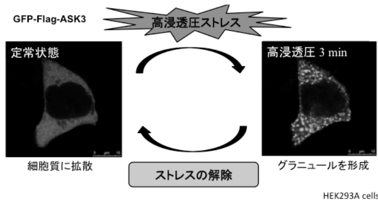
図1 ASK3は高浸透圧ストレスに応じて迅速かつ可逆的にグラニューールを形成する
