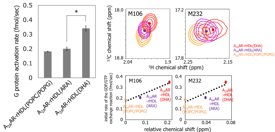
図 2. (左)各脂質組成の A_{2A}AR -rHDL の G タンパク質活性化能。 p < 0.01 。(右上)各脂質組成の A_{2A}AR -rHDL における、M106 および M232 の NMR シグナル。(右下)各脂質組成の A_{2A}AR -rHDL における、G タンパク質活性化能と M106 および M232 の化学シフトの相関。
