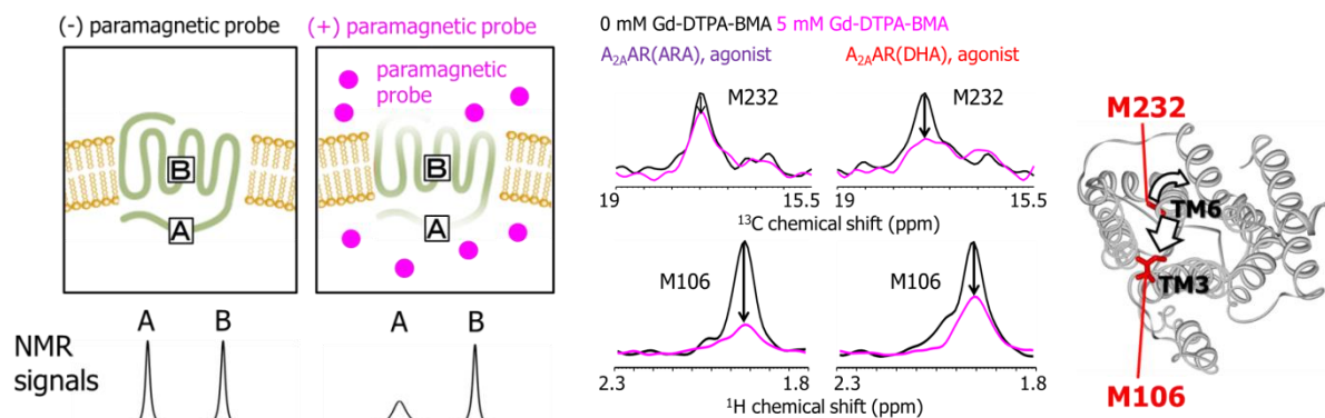
図 3. (左)solvent PRE 実験の概要。試料に常磁性試薬 Gd-DTPA-BMA を添加すると、Gd-DTPA-BMA から距離に依存して NMR シグナルが広幅化して、強度減少する。したがって、溶媒露出度の低い残基 B と比較して溶媒露出度の高い残基 A の方が、Gd-DTPA-BMA 添加に伴い大きく強度減少する。(中) DHA 存在下および ARA 存在下における、M106 および M232 シグナルの、Gd-DTPA-BMA による強度減少の比較。(右)細胞内側から見た、DHA による A_{2A}AR の構造変化 (PDB code: 2YDV)。
