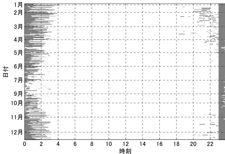
図 4 -10 提案手法における起動停止の様子 (灰色:起動、 白色:停止、 HP4.5+T200、 世帯1)
