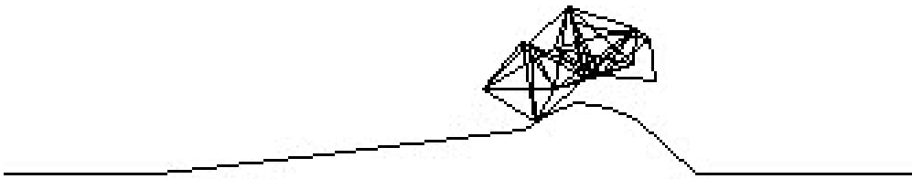
図 2-17 坂道と障害物の地形で進化させて得られたロボットの例
