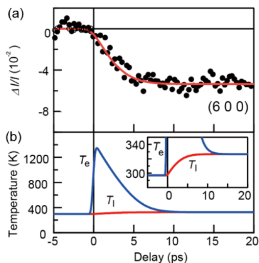
図1 (a) 金単結晶(11 nm)の(6 0 0)回折強度の時間変化。赤線は2温度モデルによるフィッティング結果。(b)得られた電子温度( T_e )および格子温度( T_l )
