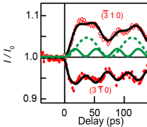
図2 VTe 2 の(-3 1 0)および(3 -1 0)回折強度の時間変化。黒実線はフィッティング結果で、緑実線および破線はフィッティング結果の振動成分。
