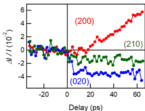
図3 \text{MoTe}_2 の(200)、(020)、(210) 回折強度の時間変化。
