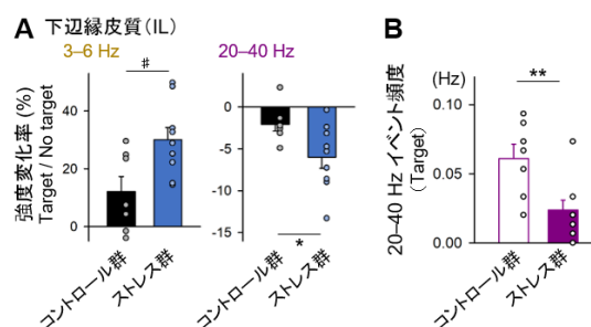
図4. 社会的回避行動時の3-6 Hzと20-40 Hzの強度変化
