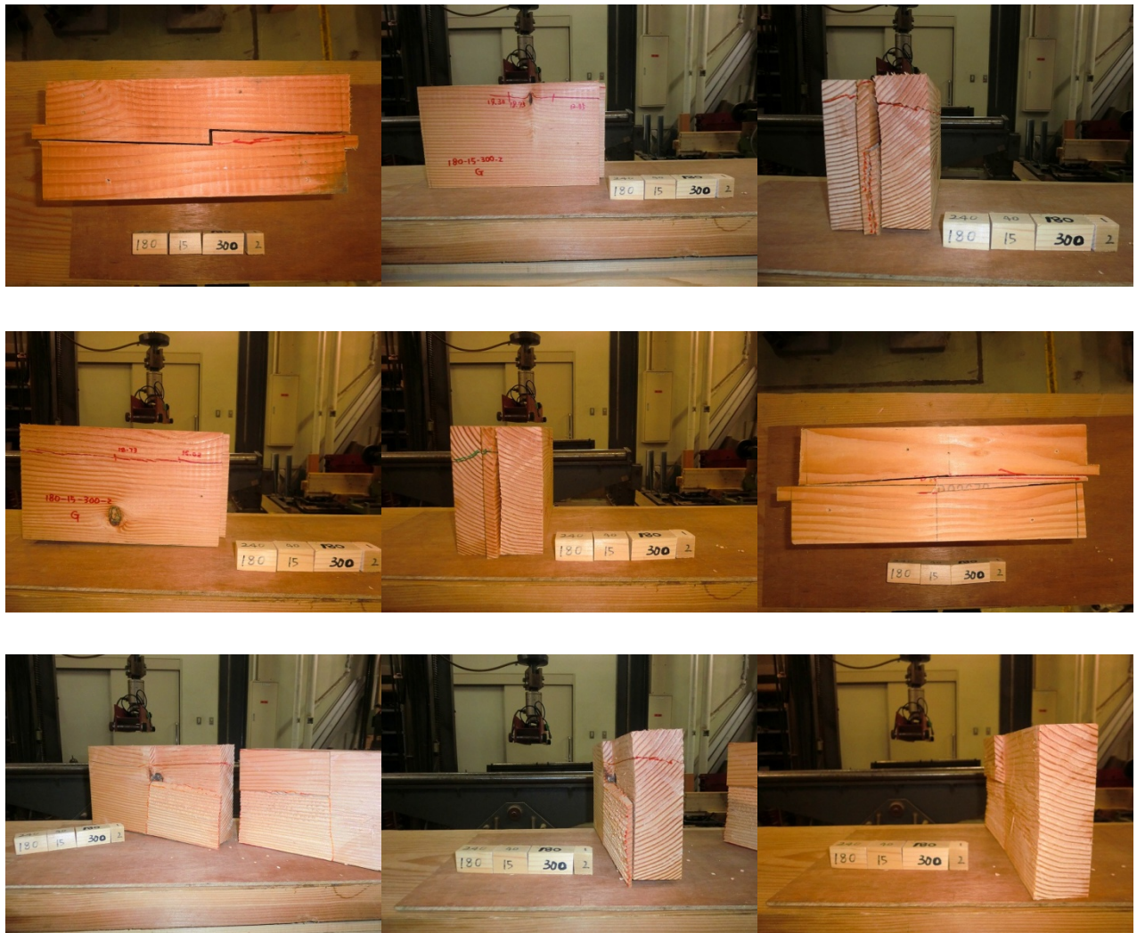
ベイマツ追掛継の4点曲げ試験データ8
