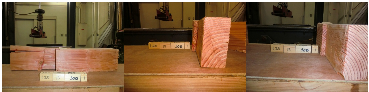
ベイマツ追掛継の4点曲げ試験データ1
