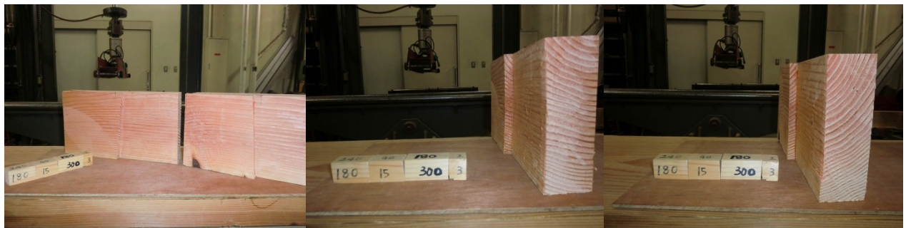
ベイマツ追掛継の4点曲げ試験データ9
