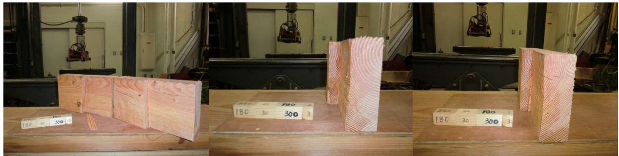
ベイマツ追掛継の4点曲げ試験データ 27
