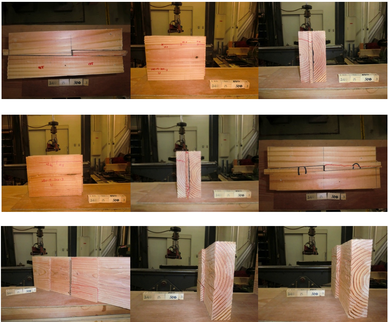
ベイツ追掛継の4点曲げ試験データ15
