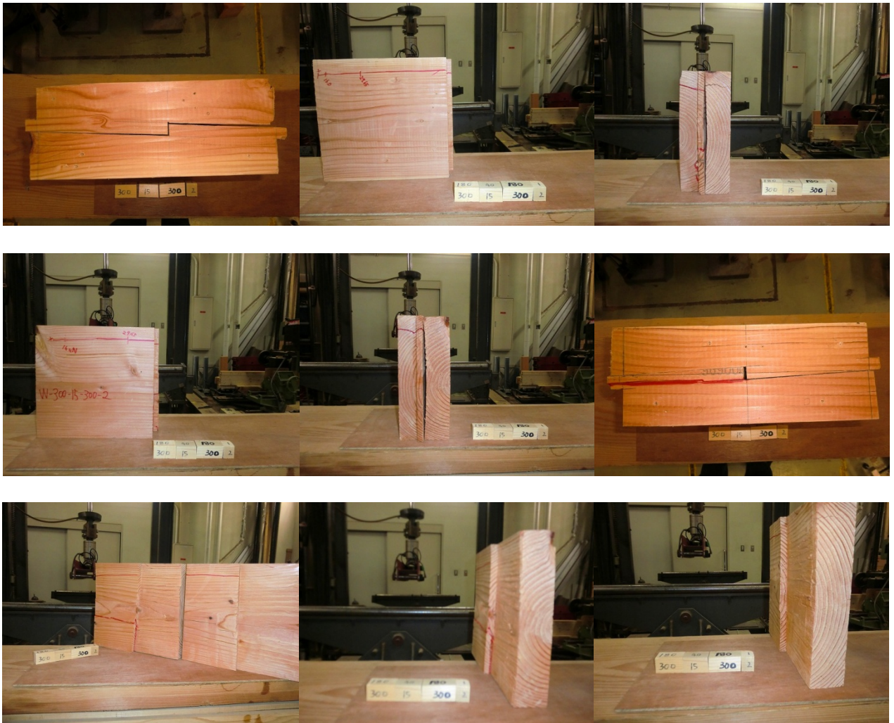
ベイツ追掛継の4点曲げ試験データ 20
