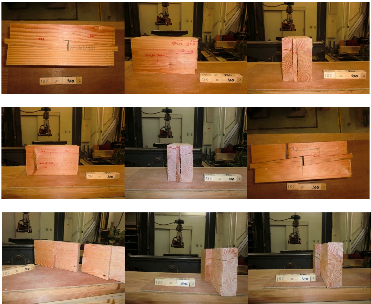
ベイツ追掛継の4点曲げ試験データ 26
