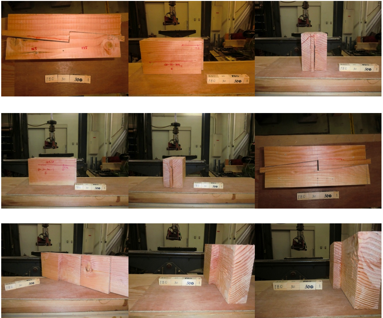
ベイマツ追掛継の4点曲げ試験データ 25
