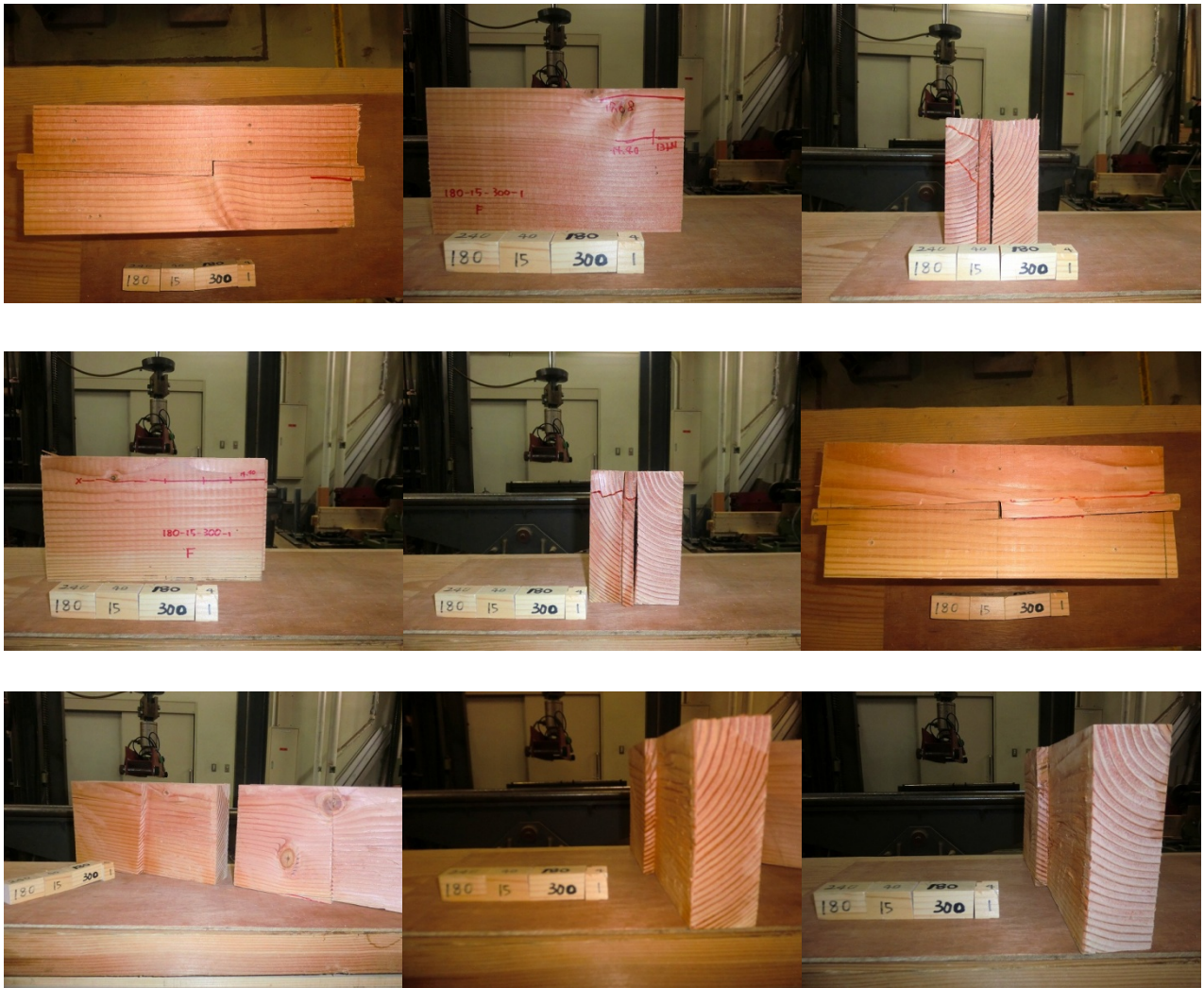
ベイマツ追掛継の4点曲げ試験データ7
