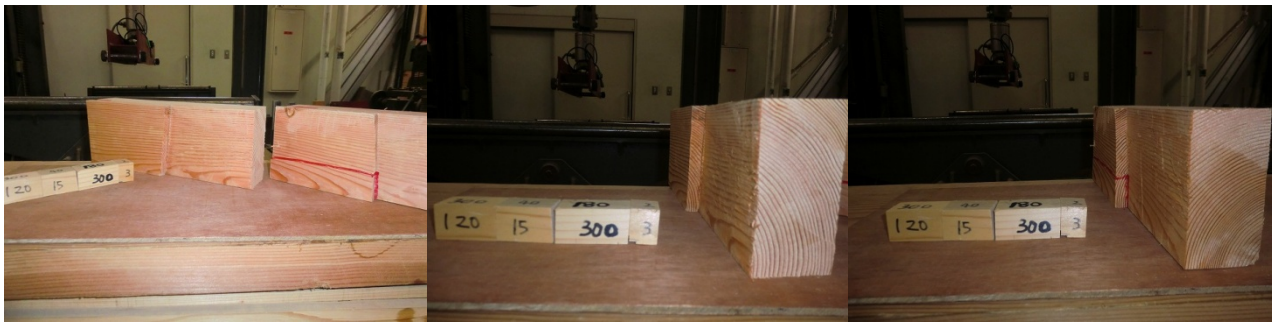
ベイマツ追掛継の4点曲げ試験データ3
