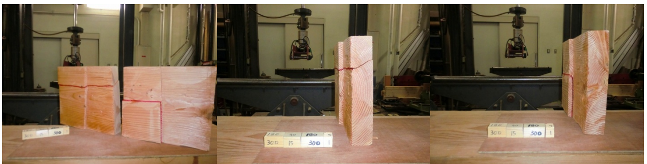
ベイマツ追掛継の4点曲げ試験データ 19
