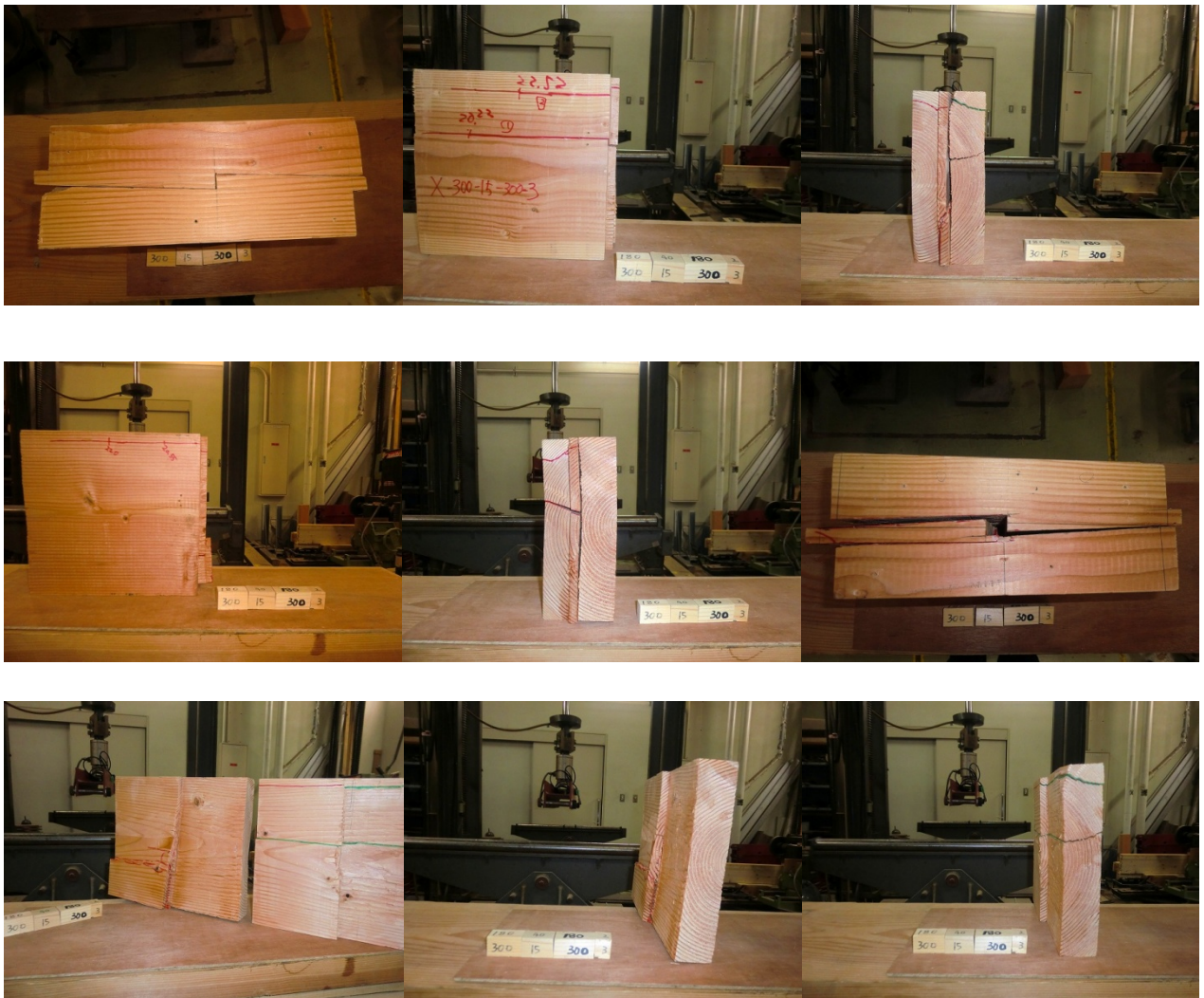
ベイツ追掛継の4点曲げ試験データ 21
