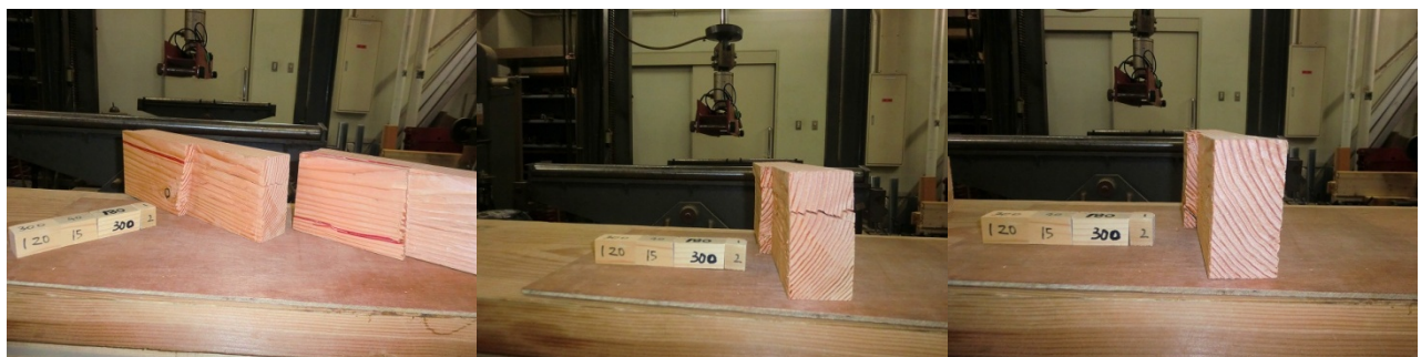
ベイマツ追掛継の4点曲げ試験データ2
