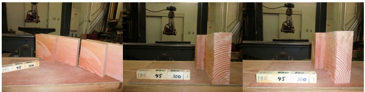
ベイツ追掛継の4点曲げ試験データ 31
