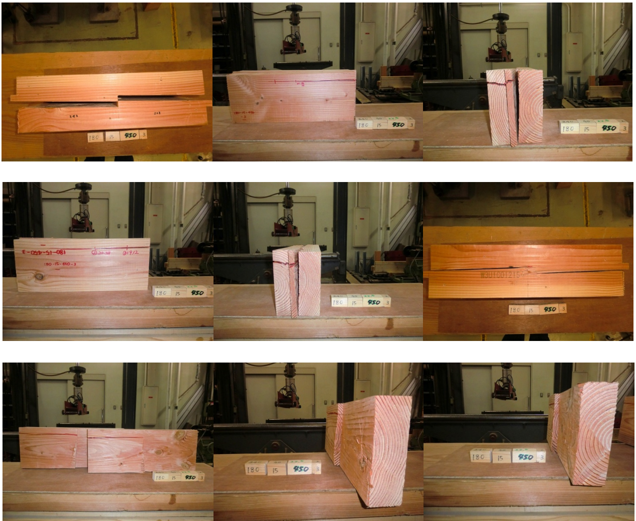
ベイツ追掛継の4点曲げ試験データ 51
