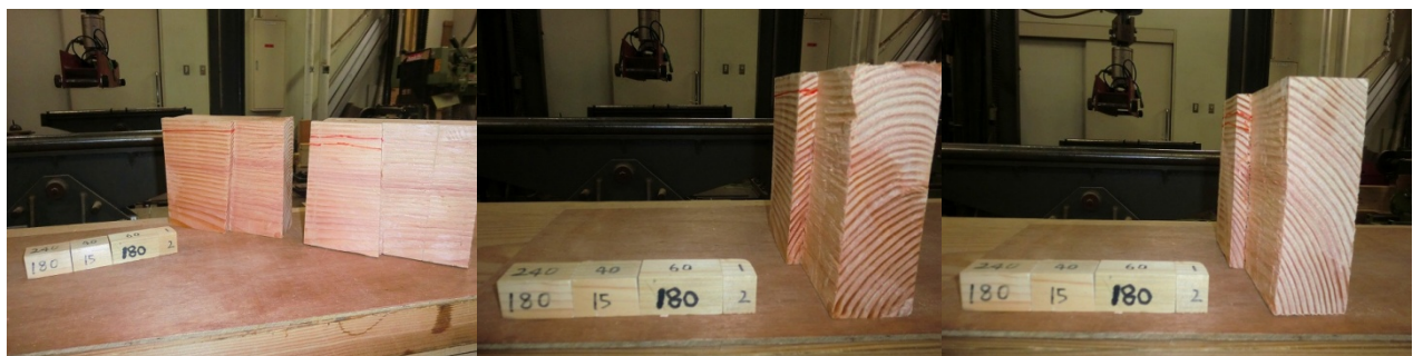
ベイマツ追掛継の4点曲げ試験データ 44
