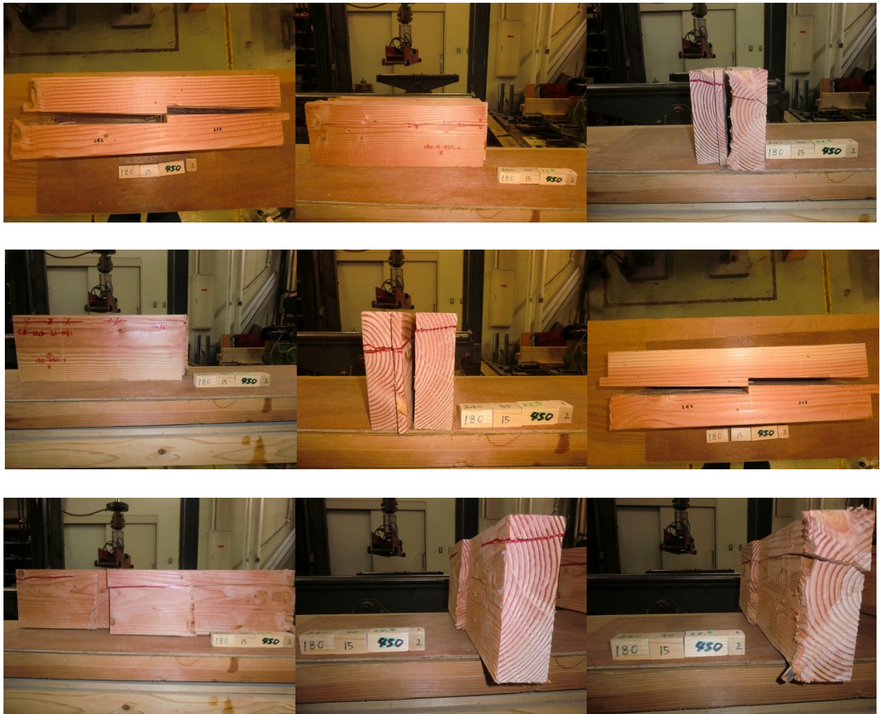
ベイマツ追掛継の4点曲げ試験データ 50
