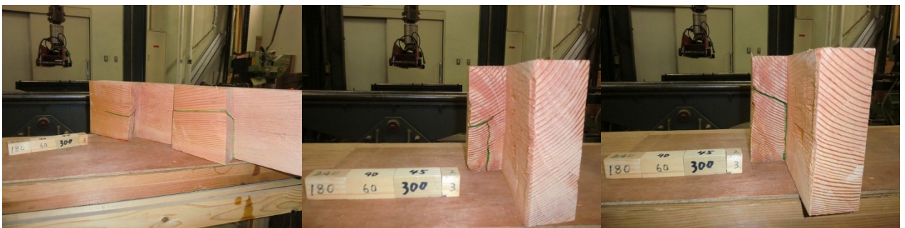
ベイツ追掛継の4点曲げ試験データ 39
