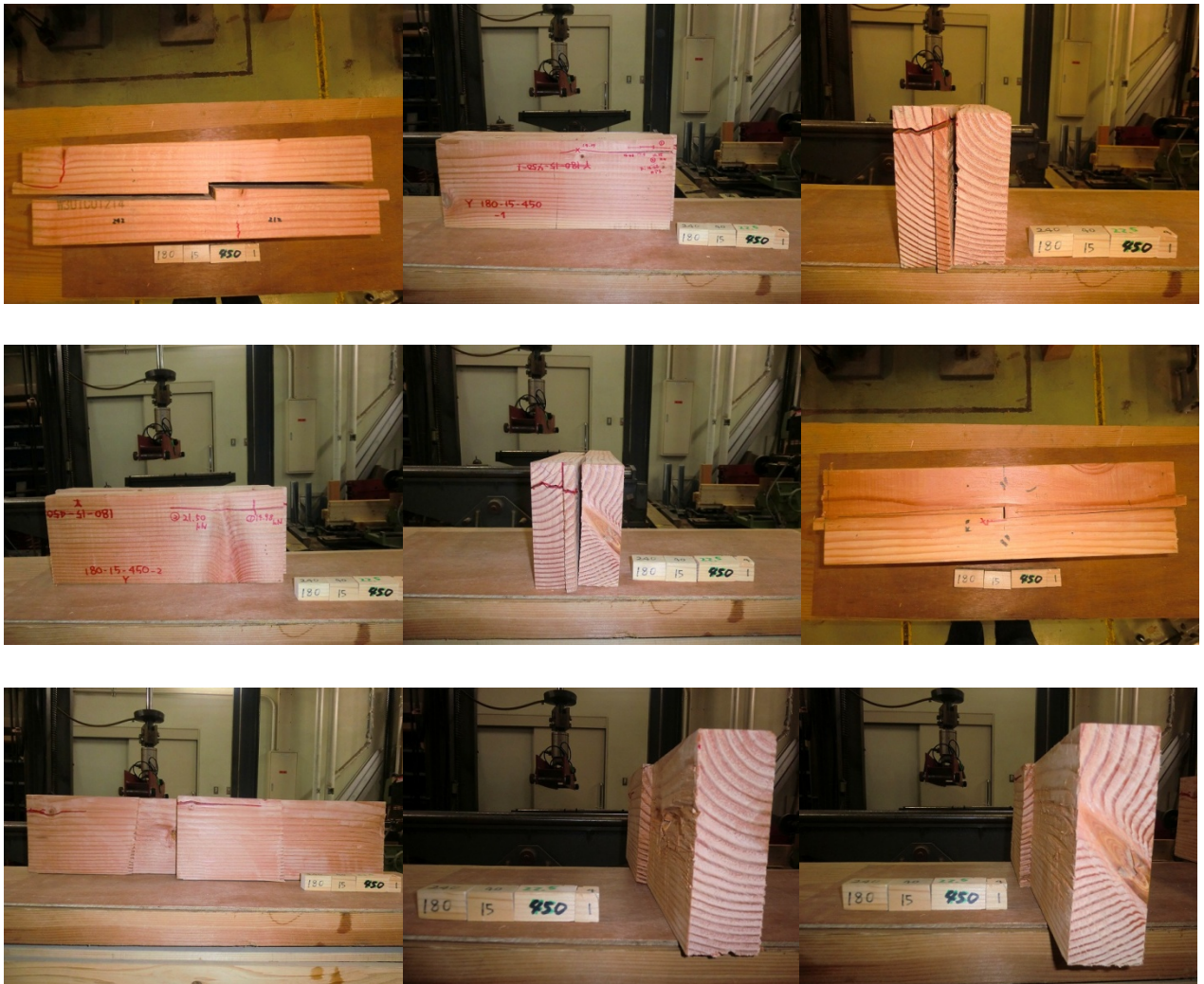
ベイマツ追掛継の4点曲げ試験データ 49
