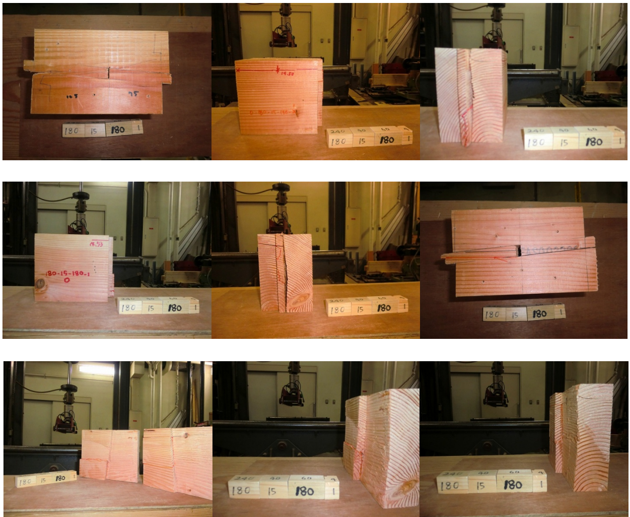
ベイマツ追掛継の4点曲げ試験データ 43
