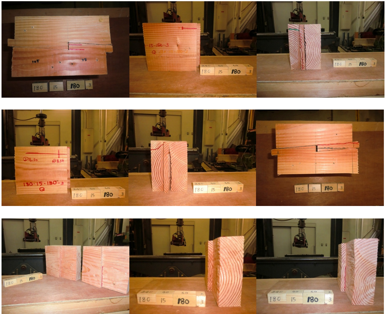
ベイマツ追掛継の4点曲げ試験データ 45
