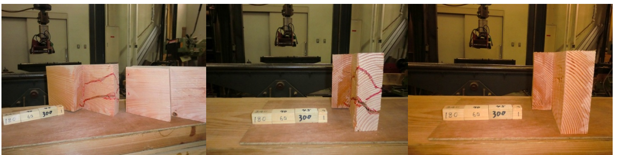
ベイマツ追掛継の4点曲げ試験データ 37
