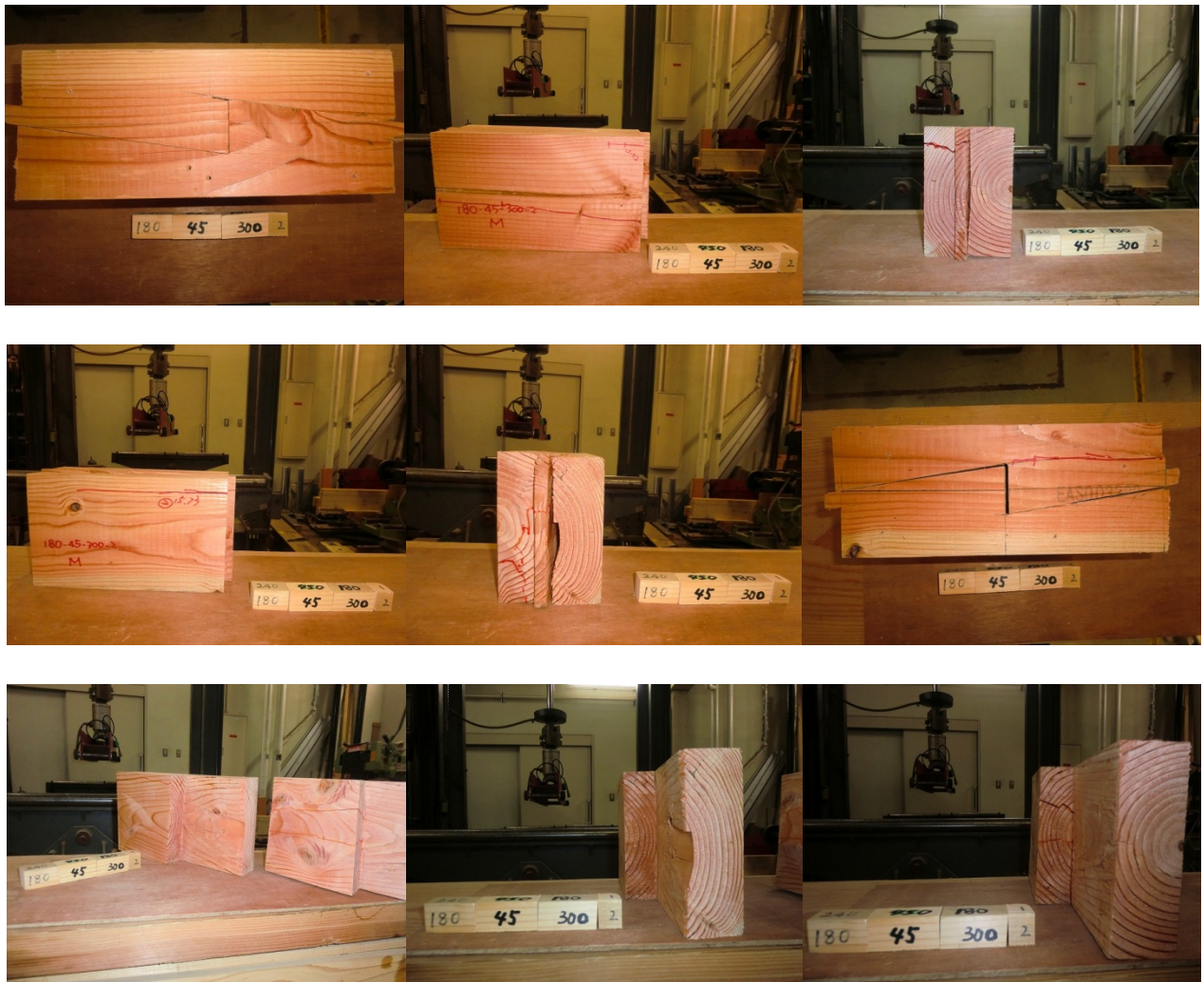
ベイツ追掛継の4点曲げ試験データ 32
