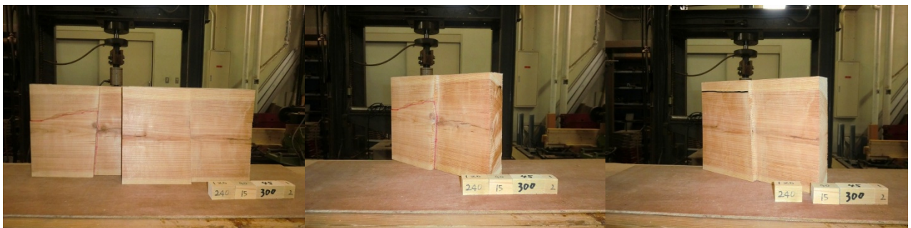
スギ追掛継の4点曲げ試験データ 14
