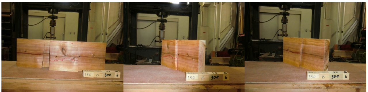
スギ追掛継の4点曲げ試験データ12
