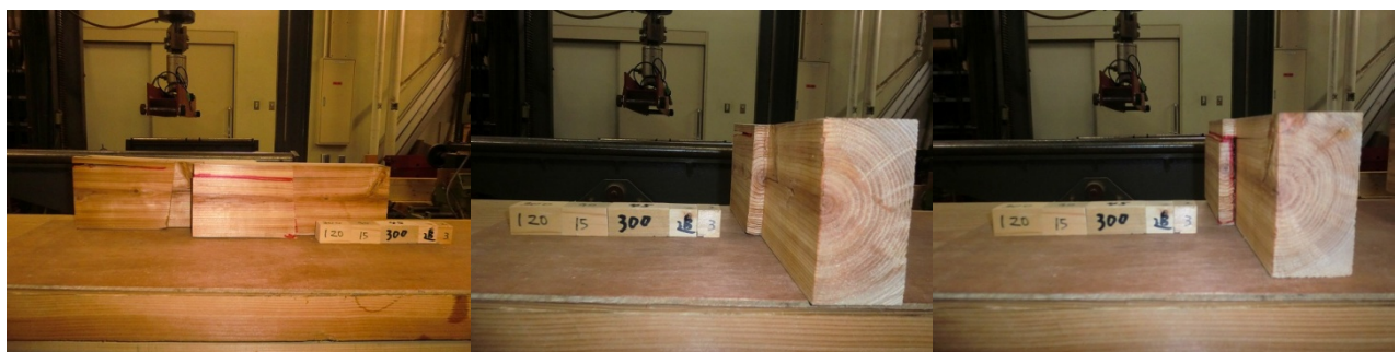
スギ追掛継の4点曲げ試験データ5
