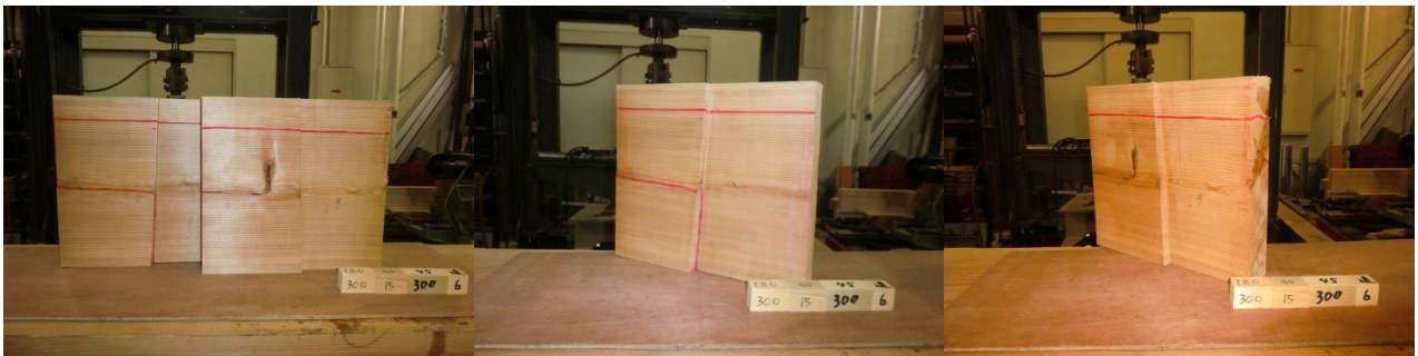
スギ追掛継の4点曲げ試験データ 24
