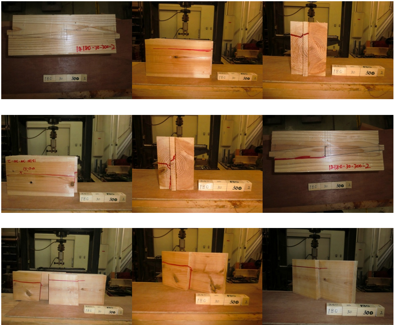
スギ追掛継の4点曲げ試験データ 26
