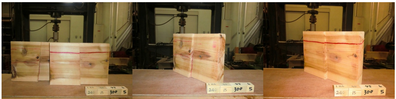
スギ追掛継の4点曲げ試験データ 17
