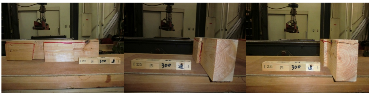
スギ追掛継の4点曲げ試験データ2
