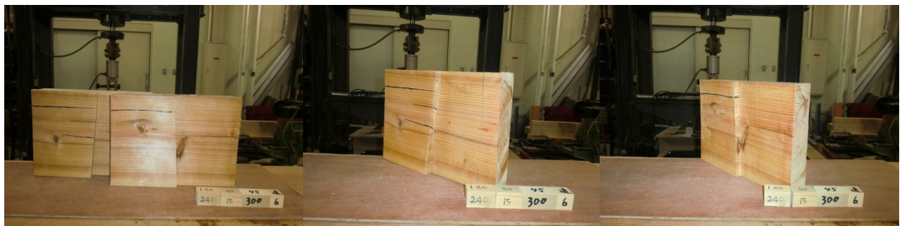
スギ追掛継の4点曲げ試験データ 18
