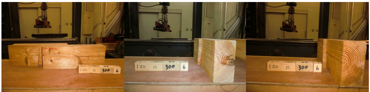
スギ追掛継の4点曲げ試験データ6
