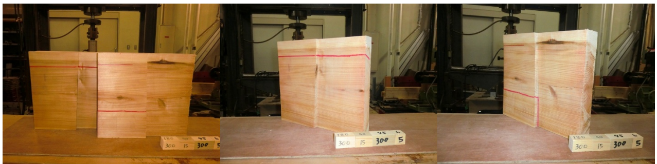
スギ追掛継の4点曲げ試験データ 23
