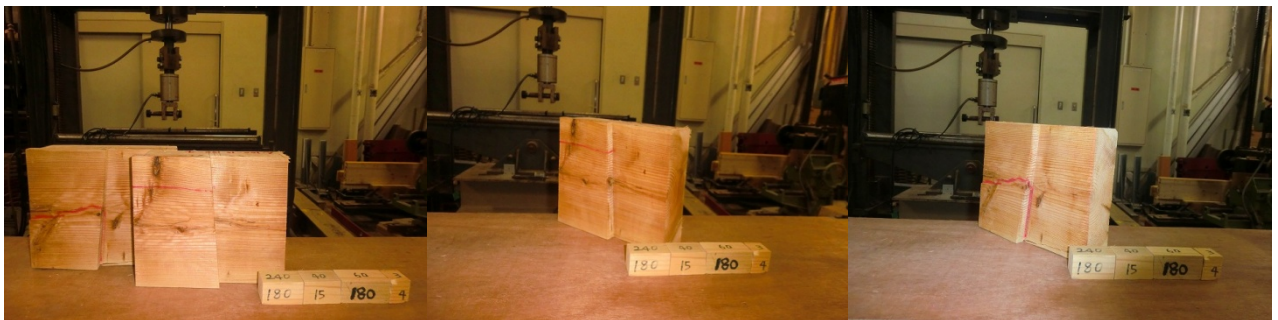
スギ追掛継の4点曲げ試験データ 46
