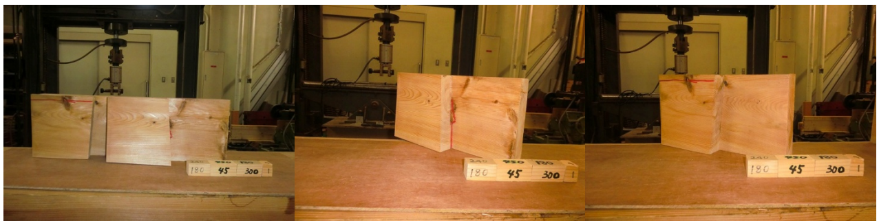
スギ追掛継の4点曲げ試験データ 31
