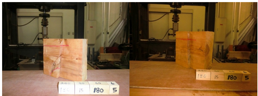
スギ追掛継の4点曲げ試験データ 47
