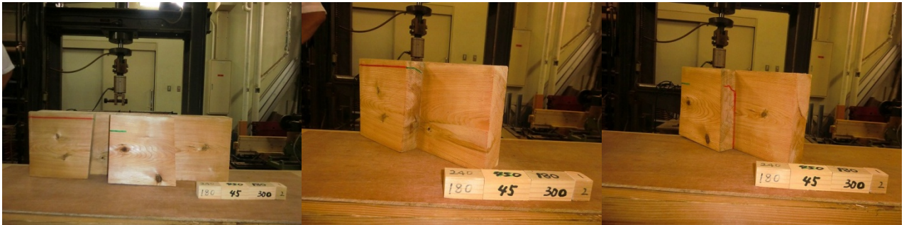
スギ追掛継の4点曲げ試験データ 32
