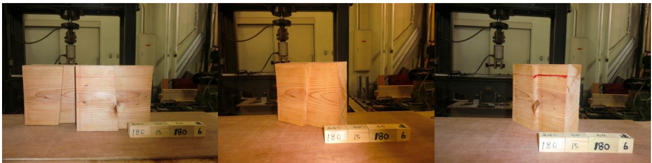
スギ追掛継の4点曲げ試験データ 48
