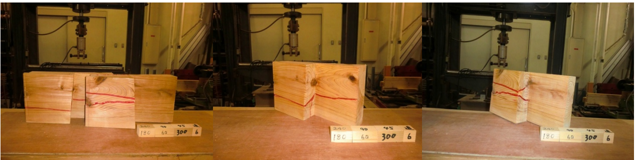
スギ追掛継の4点曲げ試験データ 42
