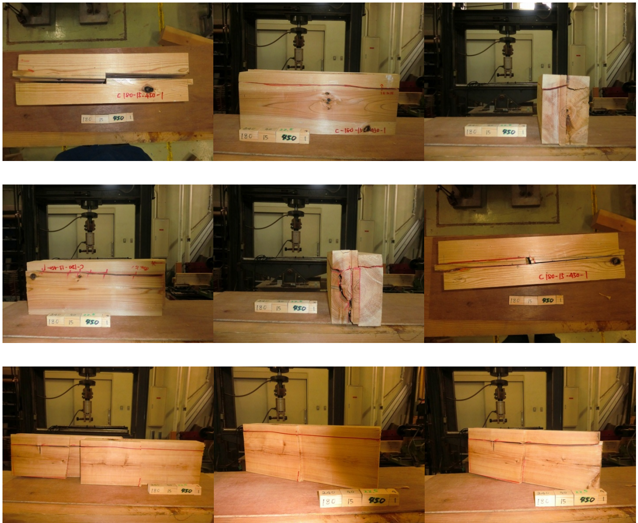
スギ追掛継の4点曲げ試験データ 49
