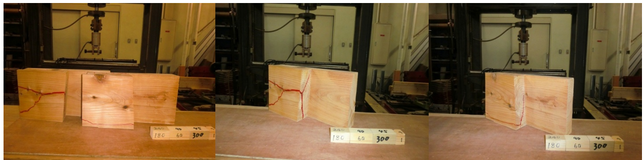
スギ追掛継の4点曲げ試験データ 37
