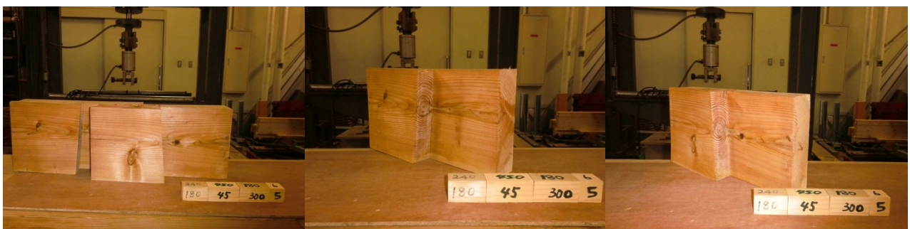
スギ追掛継の4点曲げ試験データ 35
