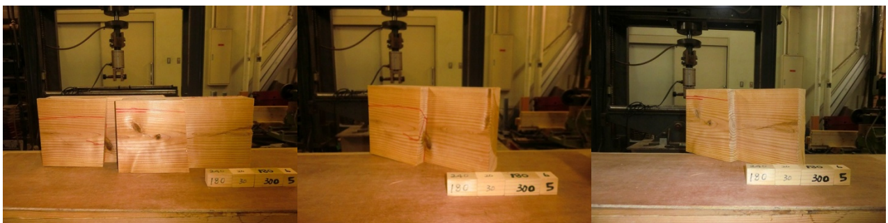
スギ追掛継の4点曲げ試験データ 29
