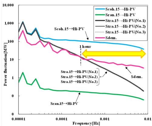
図1 PV大量導入時の出力変動推定結果
