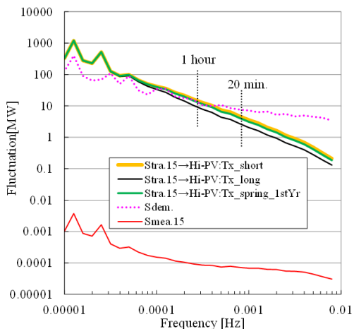
図2 遷移周期がPV大量導入時の出力変動推定結果に与える影響検討
