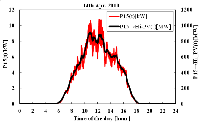
図1 PV大量導入時の出力変動推定結果
