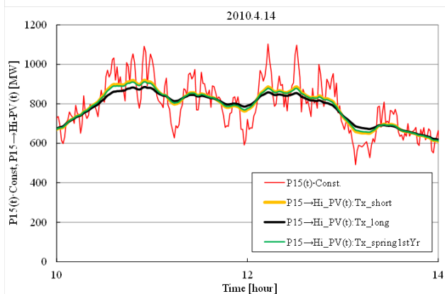
図2 遷移周期がPV大量導入時の出力変動推定結果に与える影響検討
