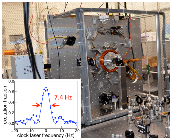
図 1: 開発した水銀光格子時計実験装置. 挿入図は時計遷移のスペクトルである.
