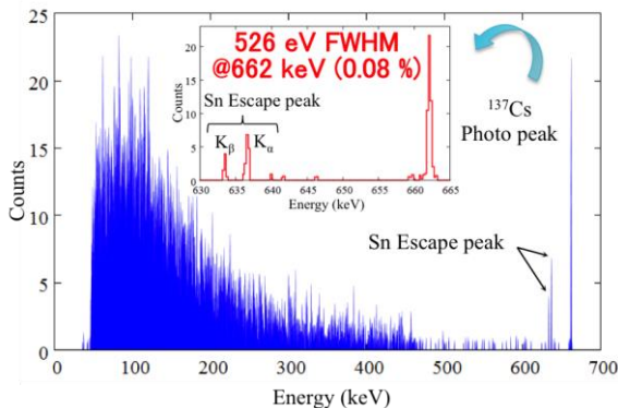
図 7. ^{137}\text{Cs} 密封放射線源から得たエネルギースペクトル
