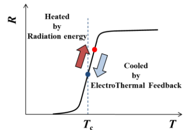
図 2. 電熱フィードバックの概念図
