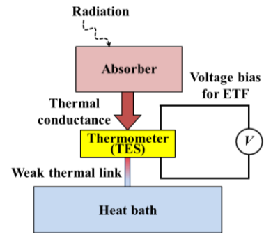
図 1. TES の概念図
