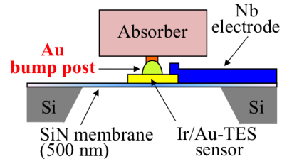
図 3. Au バンプポスト製 \gamma 線 TES マイクロカロリメータの断面図
